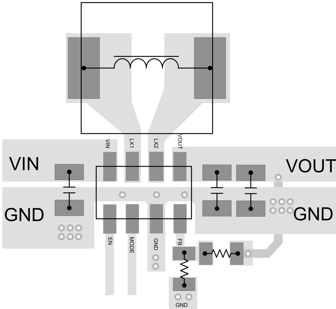
图 10-1. Layout Example
