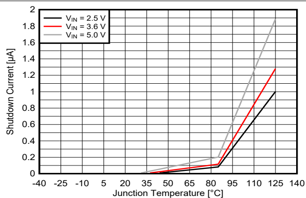
图 7-2. 关断电流与结温间的关系
