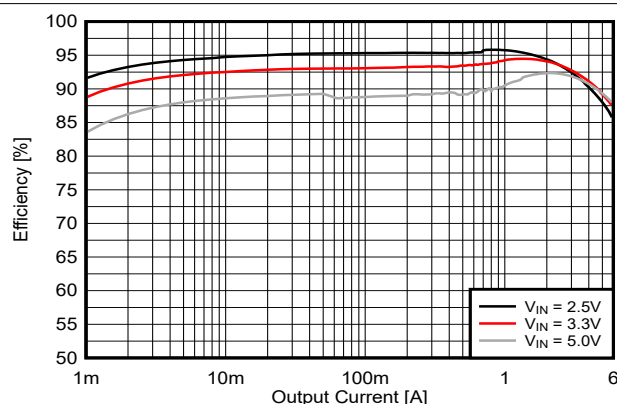
图 8-4. 1.8V 输出效率 (TPS62A04B)
