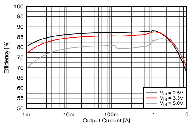
图 8-2. 0.6V 输出效率 (TPS62A04B)
