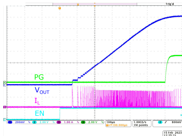
图 8-8. 在无负载条件下启动 (TPS62A04B)
