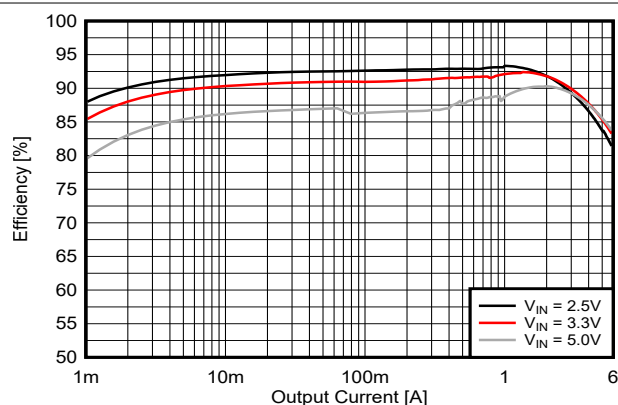
图 8-3. 1.2V 输出效率 (TPS62A04B)
