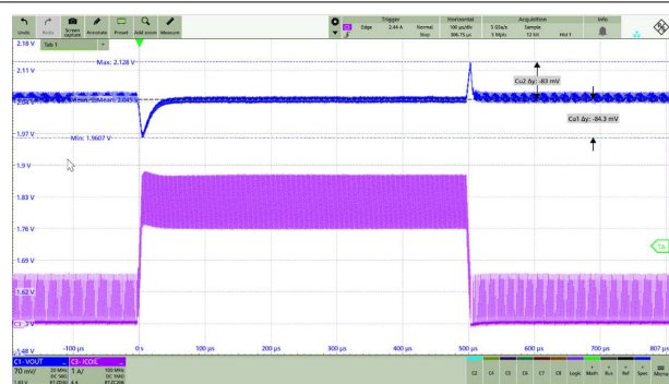
图 8-8. 在无负载条件下启动 (TPS62A04B)
