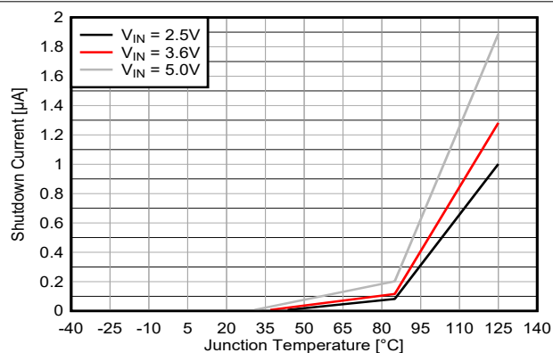
图 6-2. 关断电流与结温间的关系
