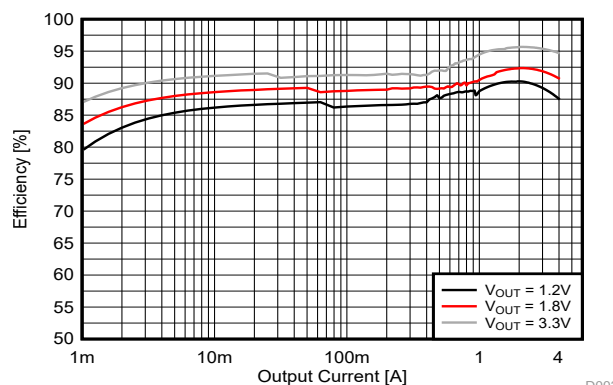
效率与输出电流间的关系曲线 ( V_{IN} = 5V 时 )
