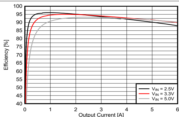
图 8-5. 1.8V 输出效率 (TPS62A04AB)
