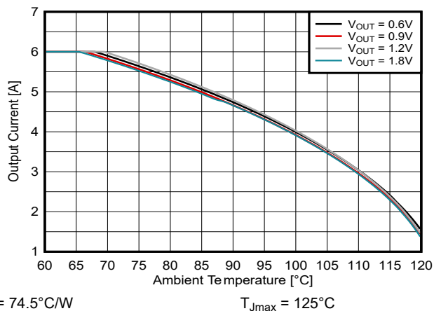
图 8-12. 基于 EVM 的安全工作区， V_{IN} = 3.3V，TPS62A04xBDRL
