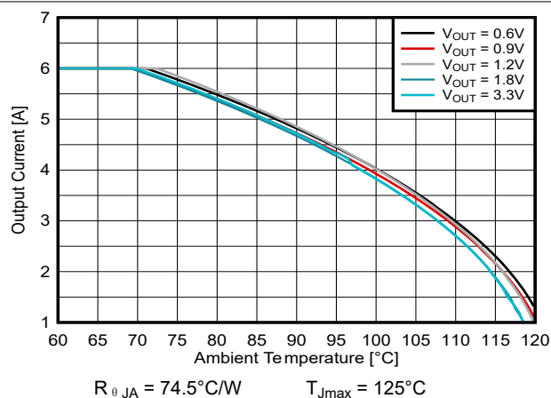
图 8-11. 基于 EVM 的安全工作区， V_{IN} = 5.0V ， TPS62A04xBDRL
