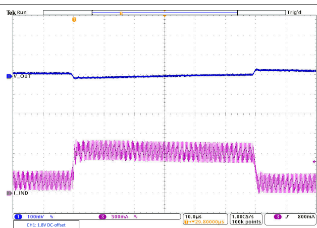
图 8-23. Load Transient
