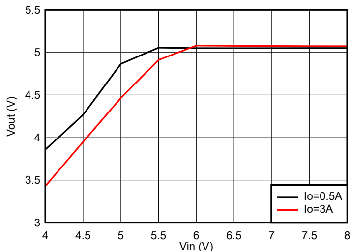
图 9-9. 总体压降特性, V_{OUT} = 5V
