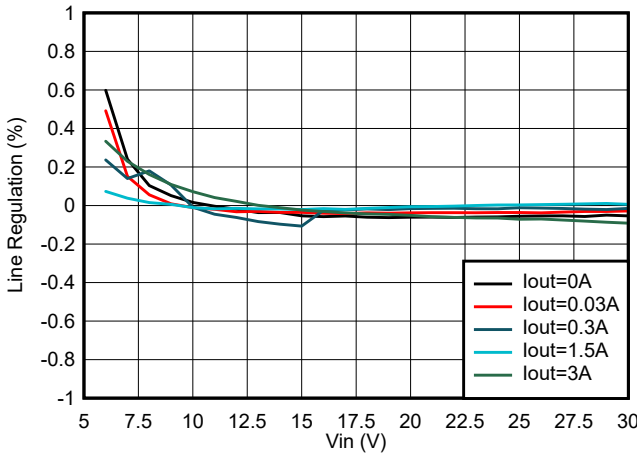
图 10-4. 线路调节
