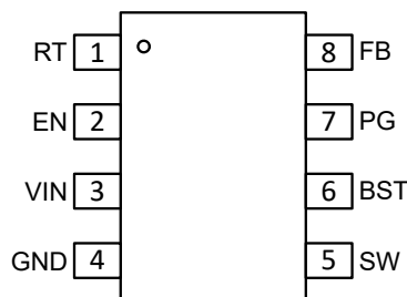
图 7-2. TPS62933P 和 TPS62933O 8 引脚 SOT583 DRL 封装 (顶视图)
