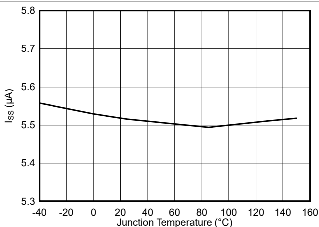
图 8-17. 软启动充电电流与结温间的关系
