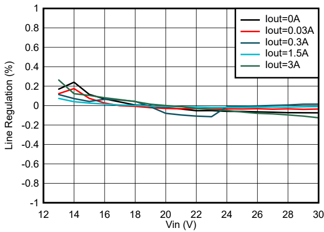
图 8-31. TPS62933 线路调节, V_{OUT} = 12\text{V} , f_{SW} = 500\text{kHz}
