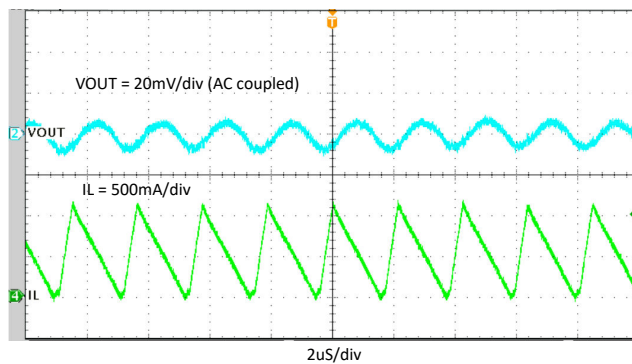
图 10-15. 稳态, I_{OUT} = 0.5A
