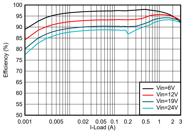
图 10-2. 效率
