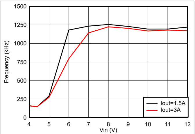
图 9-6. t_{OFF\_MIN} 时的频率折返， V_{OUT} = 5V ， f_{SW} = 1200kHz
