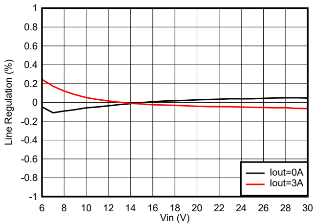
图 8-33. TPS62933F 线路调节, V_{OUT} = 5\text{V} , f_{SW} = 500\text{kHz}
