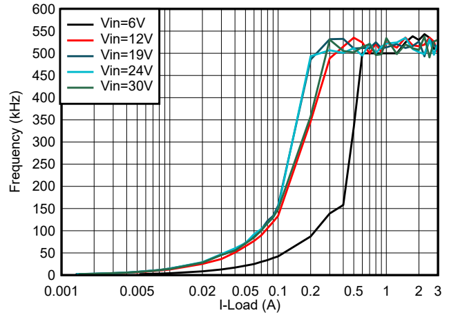
图 10-5. 开关频率与负载电流间的关系
