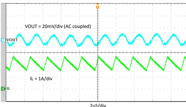
图 10-17. 稳态, I_{OUT} = 2A
