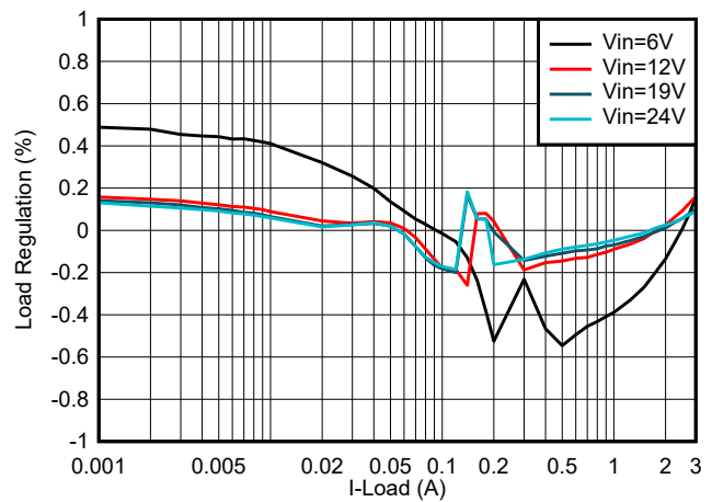
图 10-3. 负载调整率
