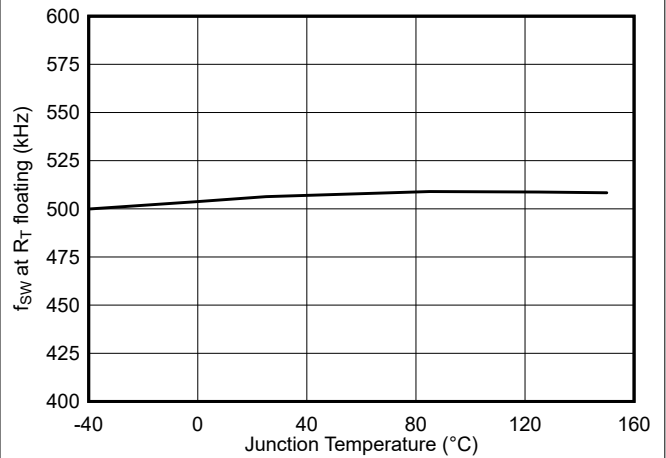
图 8-10. 开关频率 ( R_T 悬空) 与结温间的关系
