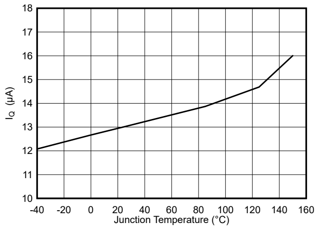
图 8-1. TPS62933 静态电流与结温间的关系
