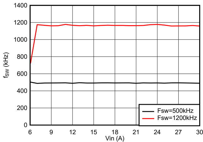
图 10-6. 开关频率与 V_{IN} 间的关系, V_{OUT} = 5V
