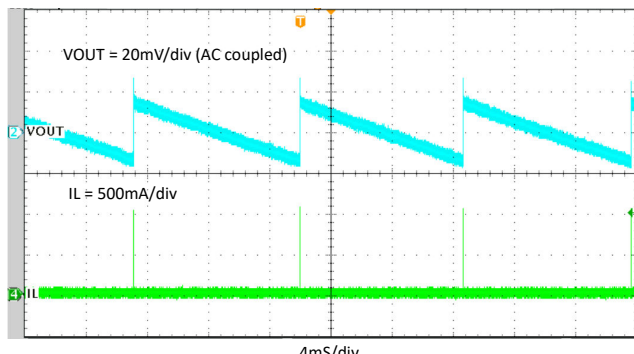
图 10-13. 稳态, I_{OUT} = 0A
