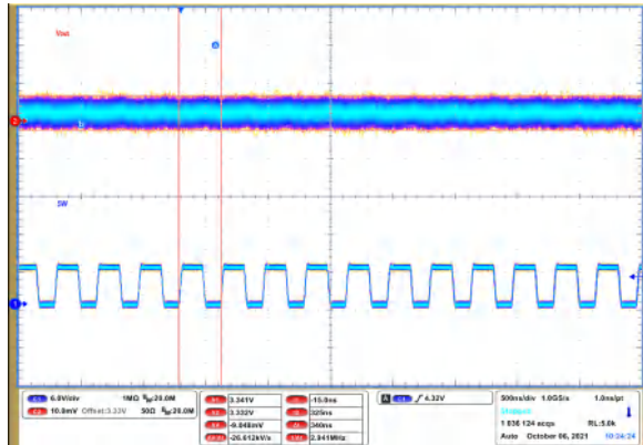
图 9-70. Output Voltage Ripple
