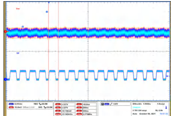
图 9-71. Output Voltage Ripple
