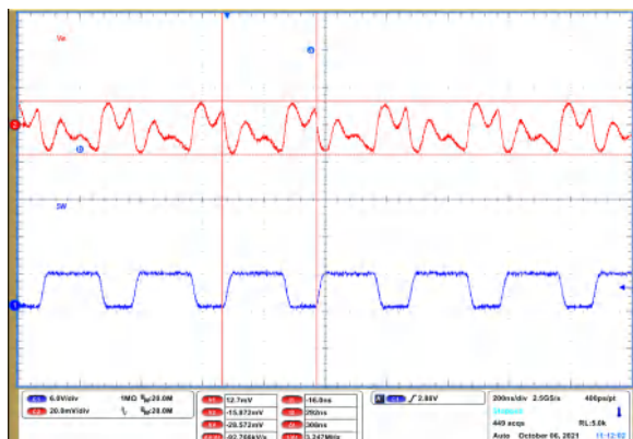
图 9-72. Output Voltage Ripple
