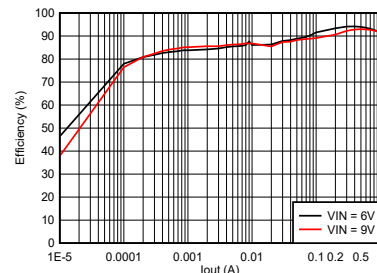
效率与输出电流间的关系 (频率为 2.5MHz, V_{\text{OUT}} = 3.3\text{V} , 自动 PFM/PWM)
