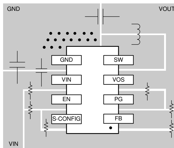
图 11-1. TPS629210E Layout
