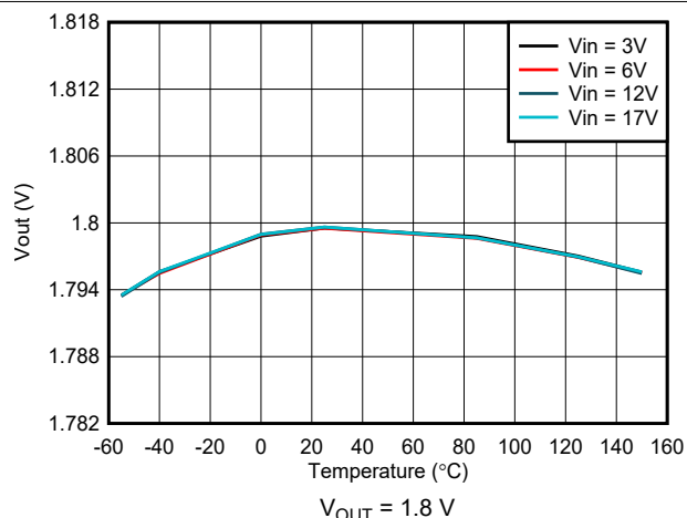
图 7-6. Output Voltage Accuracy – VSET Selected
