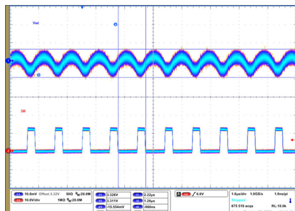
图 9-75. Output Voltage Ripple
