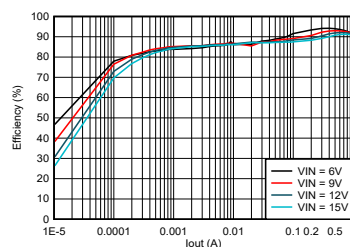
效率与输出电流间的关系 (频率为 2.5MHz, V_{\text{OUT}} = 3.3\text{V} , 自动 PFM/PWM)
