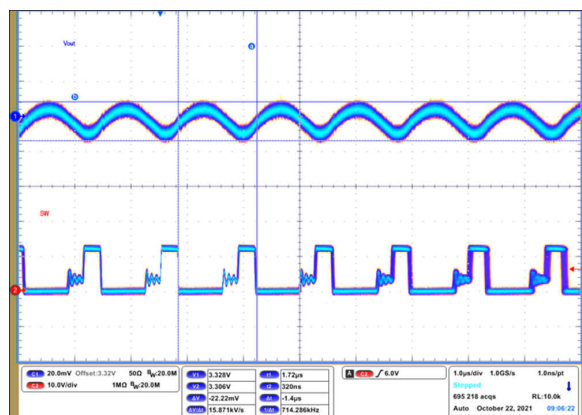
图 9-74. Output Voltage Ripple
