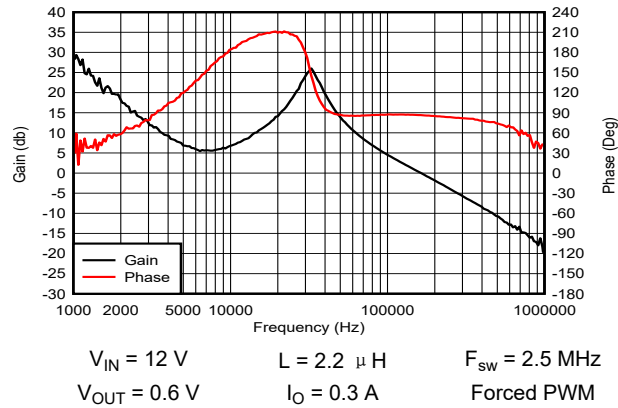
图 9-80. Bode Plot
