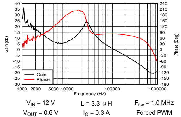
图 9-81. Bode Plot
