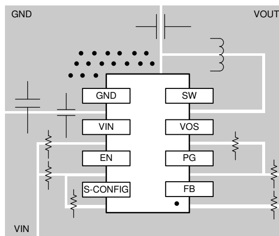
图 11-1. TPS629203-Q1 Layout
