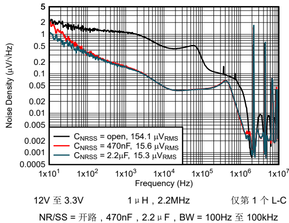
图 5-17. 输出噪声密度与频率间的关系
