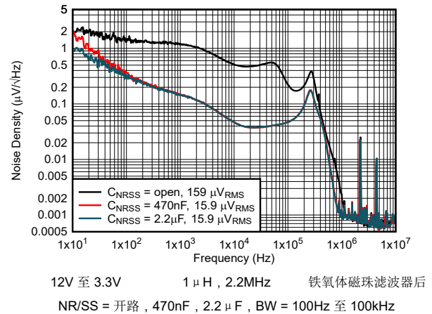
图 5-18. 输出噪声密度与频率间的关系
