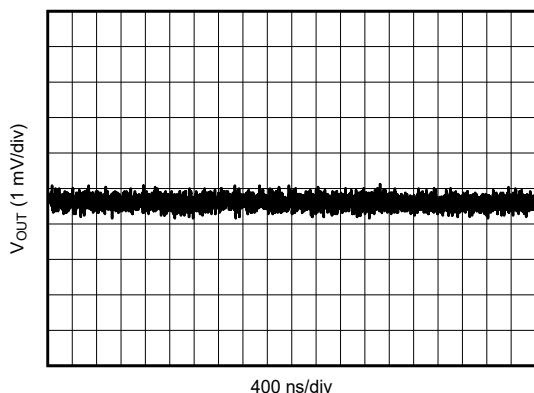
图 5-11. 第 2 个 L-C 滤波器之后的 V_{OUT} 纹波
