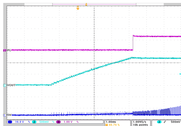
图 7-2. 启动
