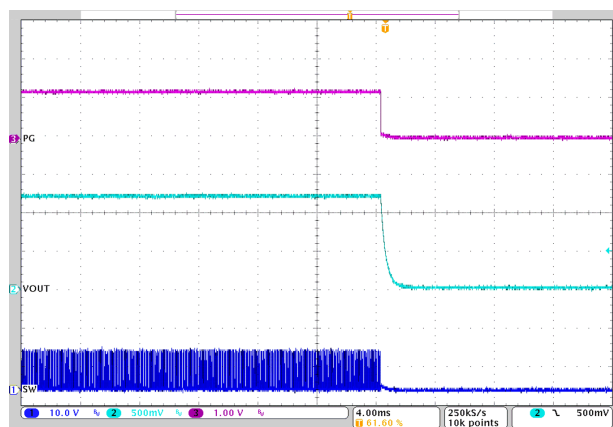
图 7-3. 关断
