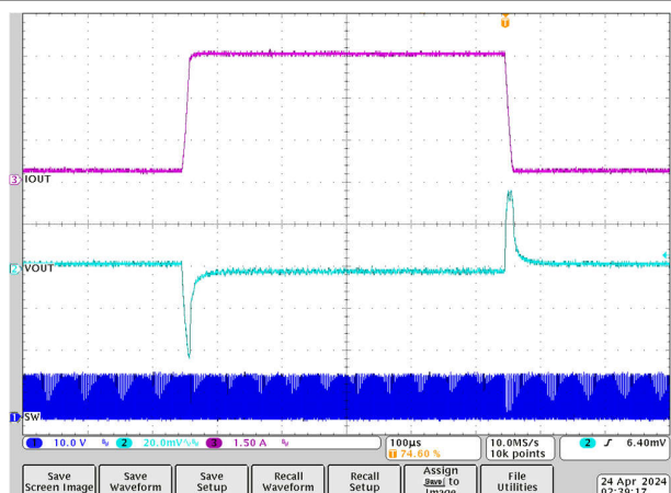
300mA 至 4.5A 至 300mA 12V 至 1.2V 1 \mu H, 1MHz 第 2 个 L-C 后 图 7-9. 负载瞬态
