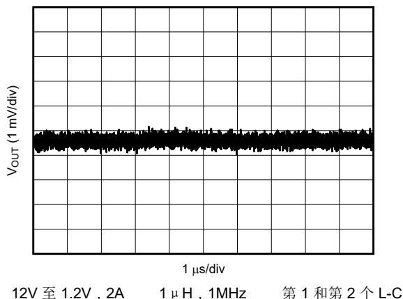
图 5-3. 第 2 个 L-C 滤波器之后的 V_{OUT} 纹波
