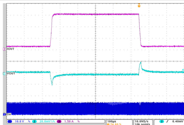
300mA 至 4.5A 至 300mA 12V 至 1.8V 1 \mu H, 1MHz 仅第 1 个 L-C 图 7-10. 负载瞬态
