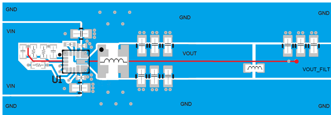
图 7-15. 使用第二个 L-C 滤波器的设计的建议布局
