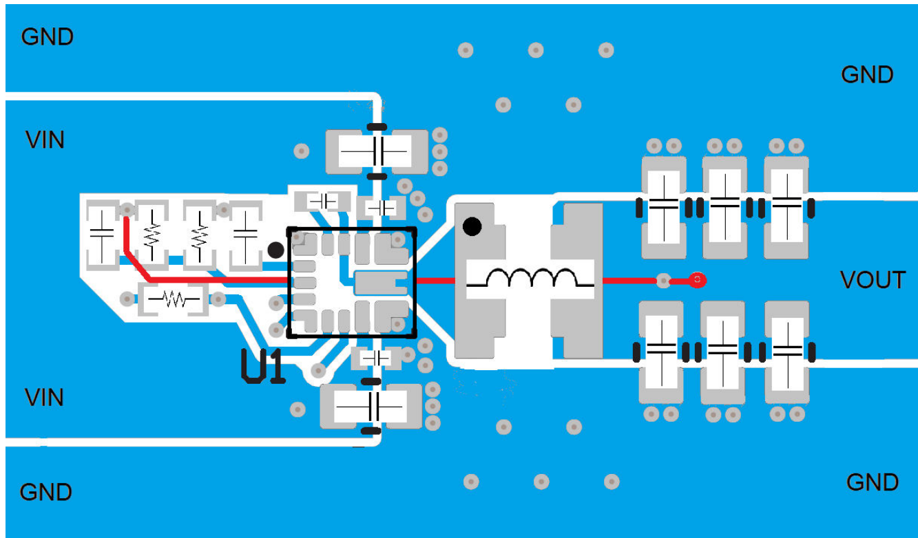
图 7-14. 单个 L-C 滤波器的建议布局
