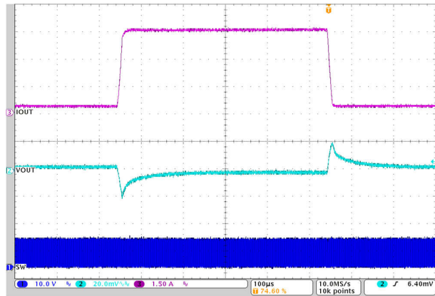
300mA 至 4.5A 至 300mA 12V 至 3.3V 1 \mu H, 2.2MHz 仅第 1 个 L-C 图 7-12. 负载瞬态
