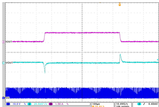
30mA 至 1.5A 至 30mA 12V 至 1.2V 1 \mu H, 1MHz 第 2 个 L-C 后 图 7-7. 负载瞬态
