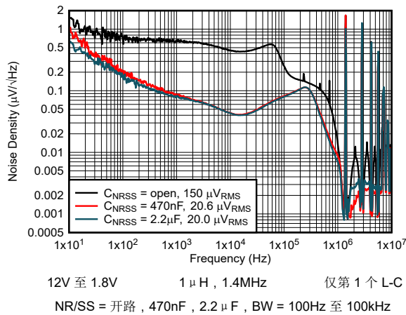
图 5-15. 输出噪声密度与频率间的关系
