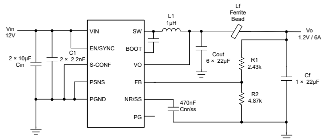
典型应用
