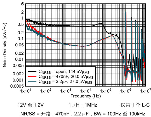
图 5-13. 输出噪声密度与频率间的关系
