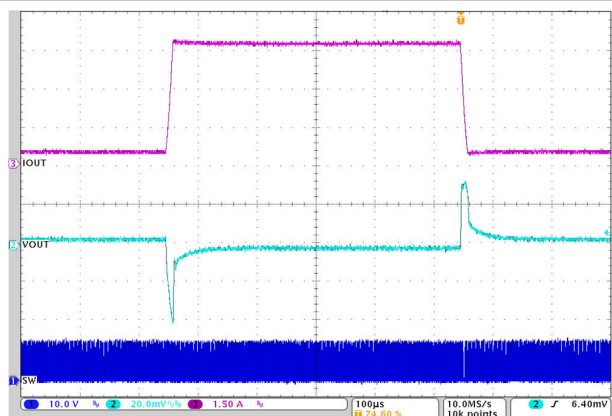
300mA 至 4.5A 至 300mA 12V 至 1.8V 1 \mu H, 1MHz 第 2 个 L-C 后 图 7-11. 负载瞬态
