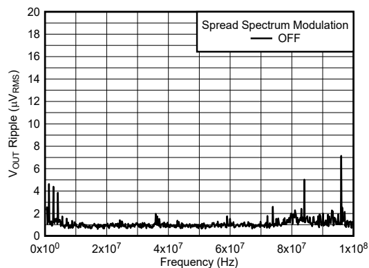
图 5-8. 第 2 个 L-C 滤波器之后的 V_{OUT} 纹波 FFT
