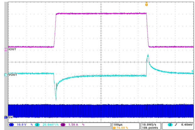
300mA 至 4.5A 至 300mA 12V 至 3.3V 1 \mu H, 2.2MHz 第 2 个 L-C 后 图 7-13. 负载瞬态
