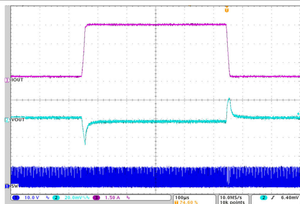
300mA 至 4.5A 至 300mA 12V 至 1.2V 1 \mu H, 1MHz 仅第 1 个 L-C 图 7-8. 负载瞬态
