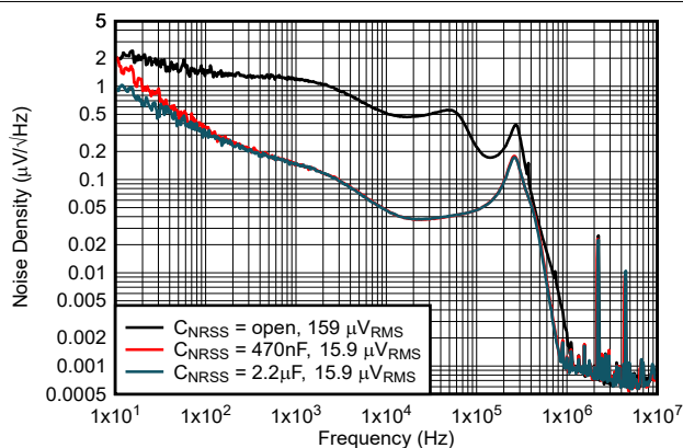
图 5-16. 输出噪声密度与频率间的关系
