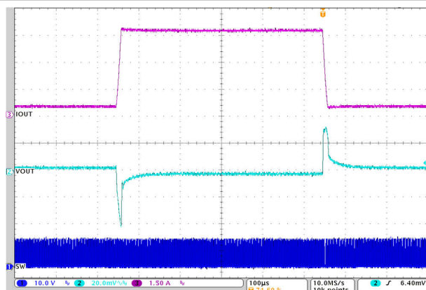
图 7-17. 负载瞬态
