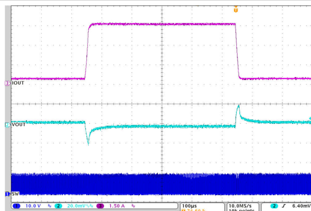
图 7-16. 负载瞬态
