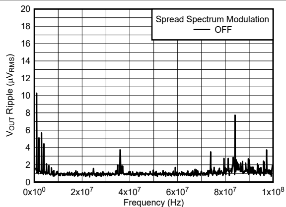
图 5-2. 第 1 个 L-C 滤波器之后的 V_{OUT} 纹波 FFT
