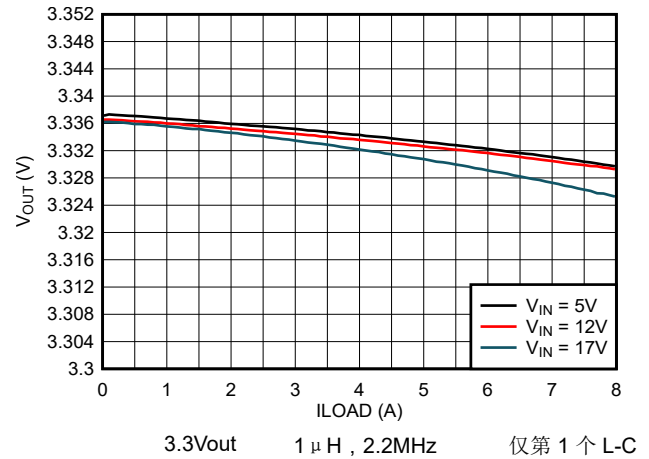
图 7-9. 输出电压与负载电流间的关系
