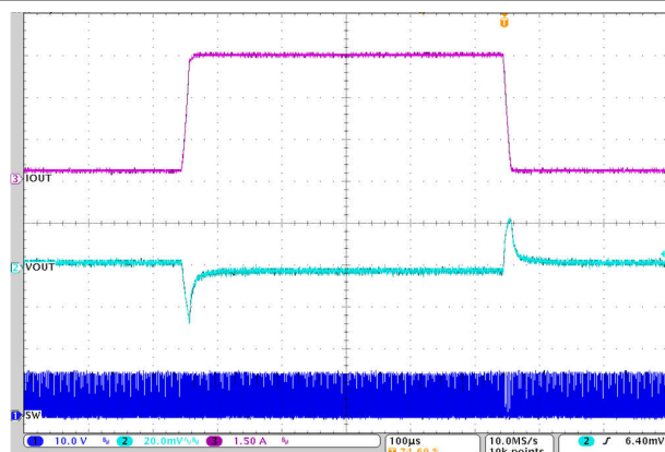
图 7-14. 负载瞬态
