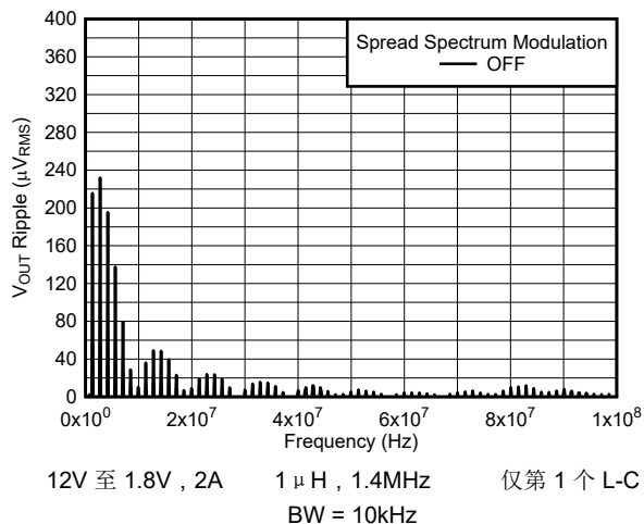
图 5-6. 第 1 个 L-C 滤波器之后的 V_{OUT} 纹波 FFT
