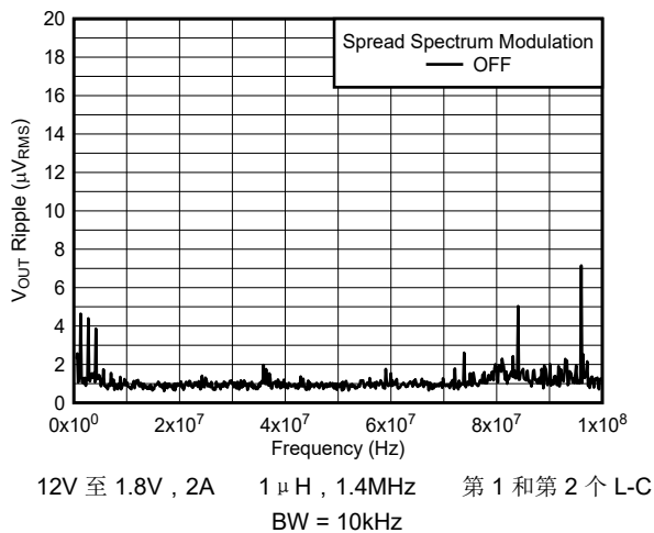
图 5-8. 第 2 个 L-C 滤波器之后的 V_{OUT} 纹波 FFT
