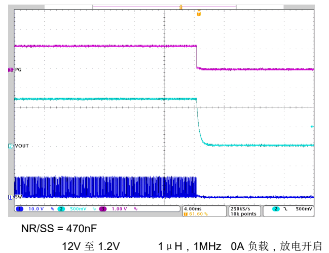
图 7-11. 关断
