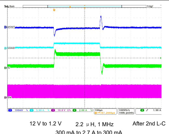
图 8-13. Load Transient
