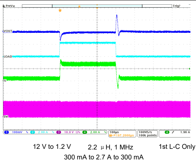
图 8-12. Load Transient
