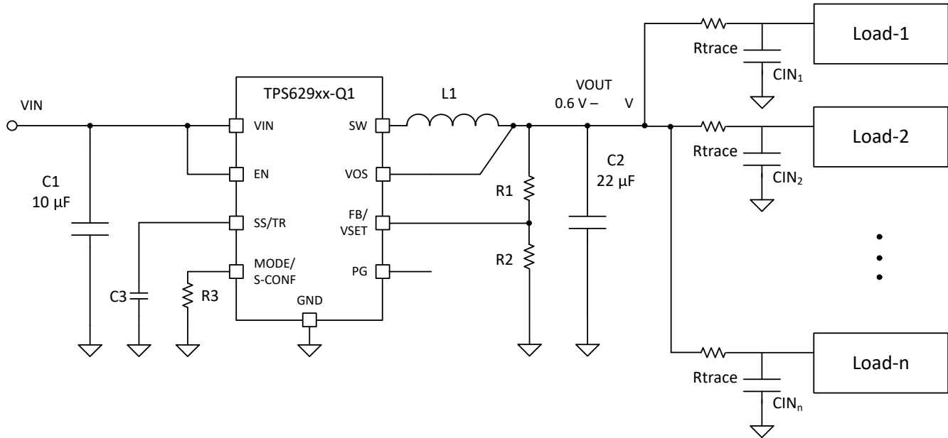
图 9-65. Multiple Loads
