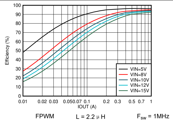
图 7-12. 效率与输出电流间的关系 V_{OUT} = 3.3V
