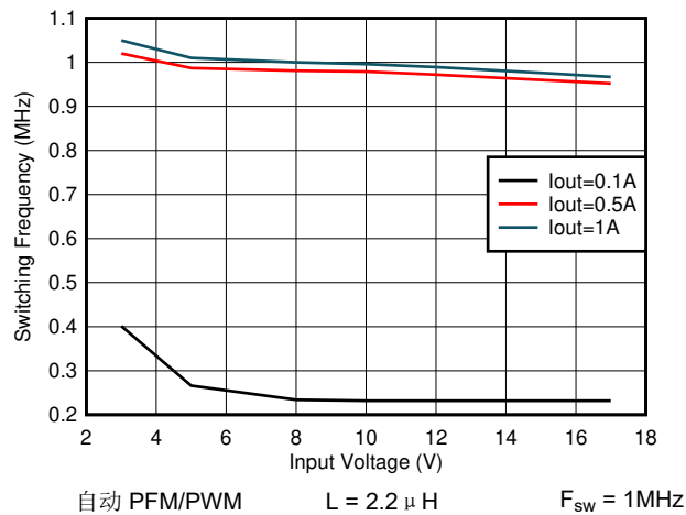
图 7-31. 开关频率与输入电压间的关系 V_{OUT} = 1.8V
