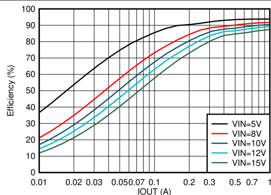
图 7-14. 效率与输出电流间的关系 V_{OUT} = 3.3V
