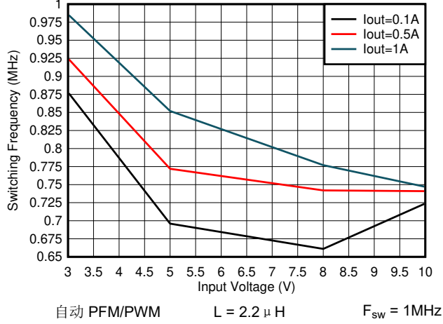
图 7-73. 开关频率与输入电压间的关系 V OUT = 0.4V
