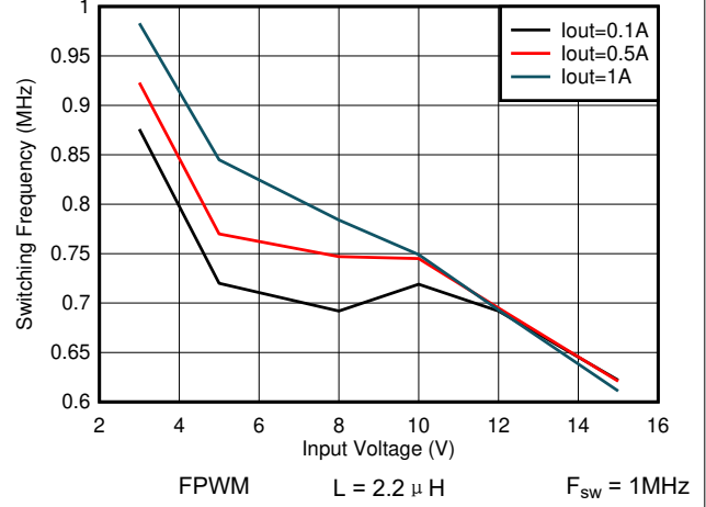
图 7-74. 开关频率与输入电压间的关系 V OUT = 0.4V
