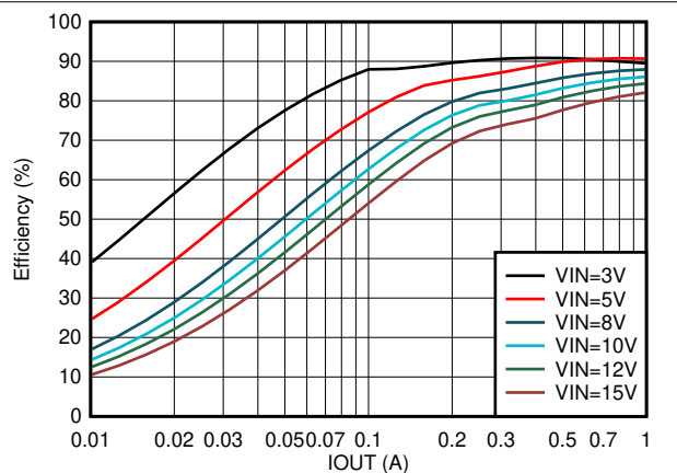
图 7-16. 效率与输出电流间的关系 V_{OUT} = 1.8V
