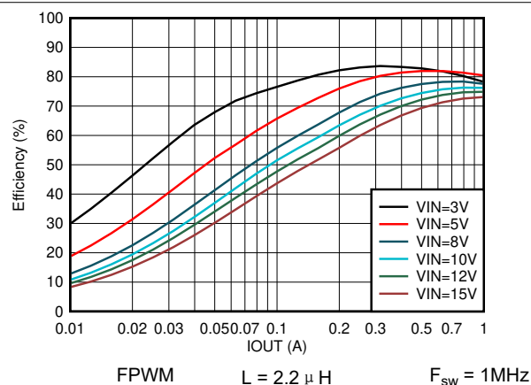
图 7-70. 效率与输出电流间的关系 V_{OUT} = 0.4V
