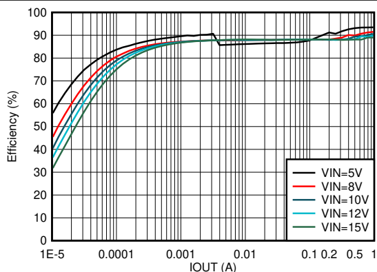
图 7-13. 效率与输出电流间的关系 V_{OUT} = 3.3V
