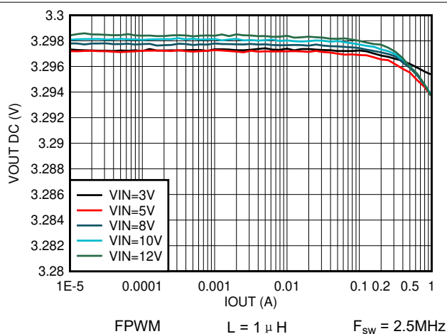
图 7-39. 输出电压与输出电流间的关系 V_{OUT} = 3.3V
