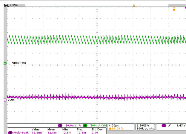
图 7-50. 输出电压纹波
