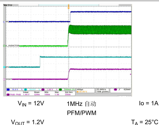
图 7-42. 启动时序
