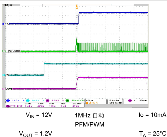
图 7-41. 启动时序
