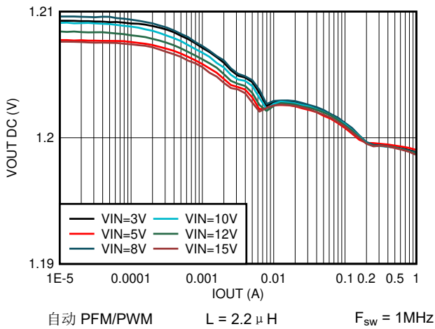
图 7-77. 输出电压与输出电流间的关系 V OUT = 1.2V
