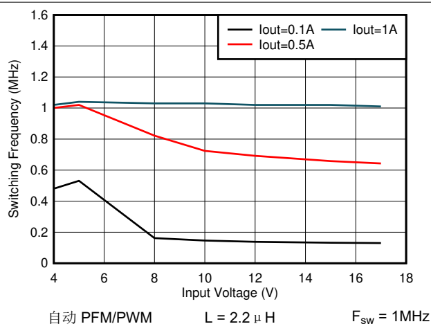
图 7-27. 开关频率与输入电压间的关系 V_{OUT} = 3.3V
