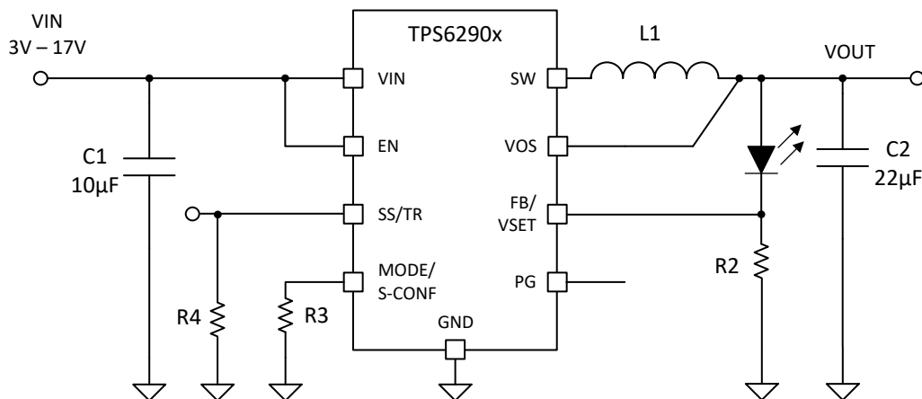
图 7-81. 单电源 LED 电源
