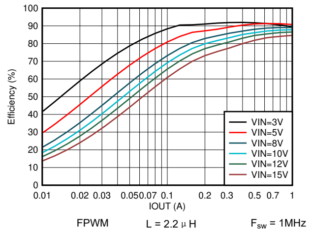
图 7-20. 效率与输出电流间的关系 V_{OUT} = 1.2V
