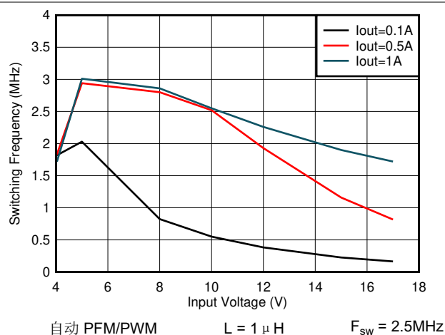
图 7-29. 开关频率与输入电压间的关系 V_{OUT} = 3.3V
