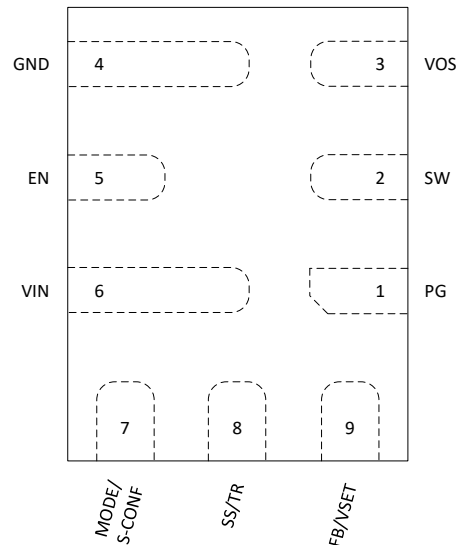
图 4-1.9 引脚 RPJ VQFN 封装 ( 顶视图, 器件引脚朝下 )
