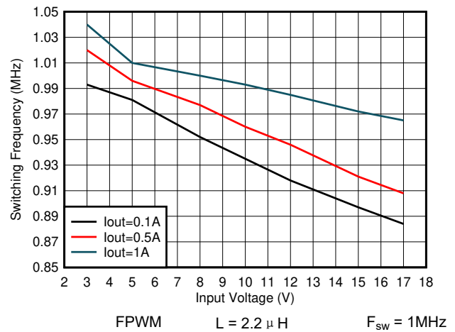
图 7-32. 开关频率与输入电压间的关系 V_{OUT} = 1.8V
