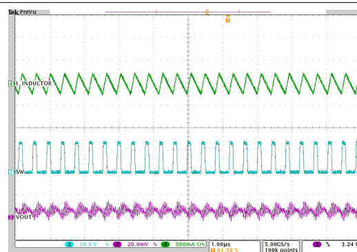
图 7-52. 输出电压纹波
