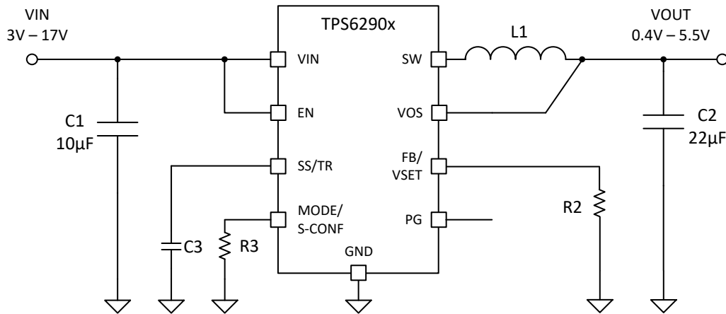
图 7-66. 典型应用电路 (VSET)
