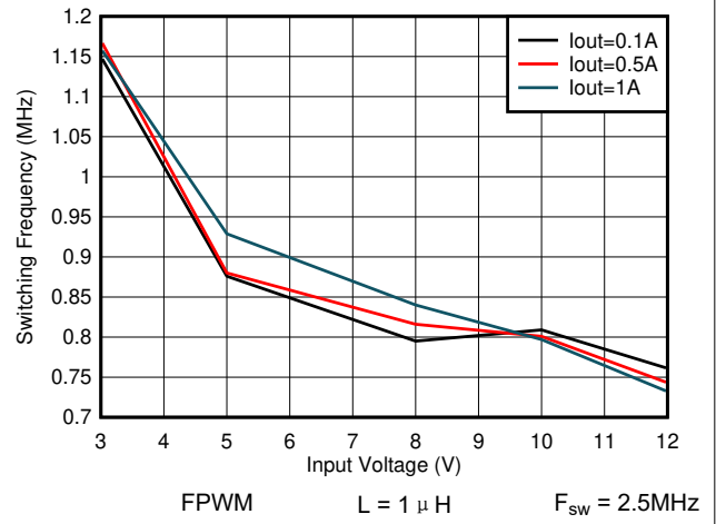
图 7-76. 开关频率与输入电压间的关系 V OUT = 0.4V
