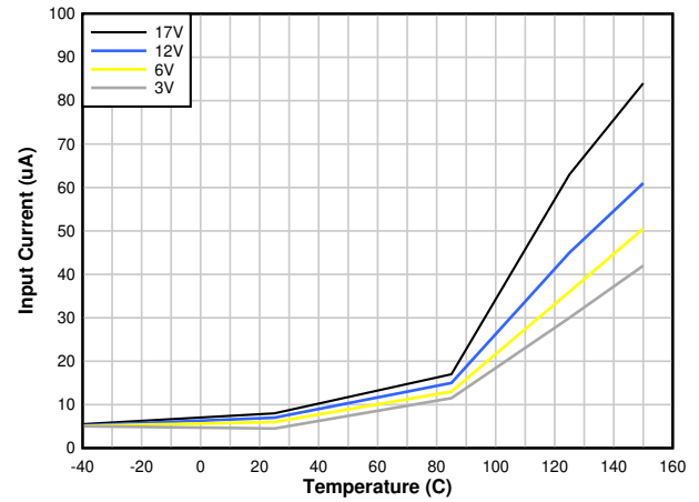
图 5-2. 最大静态电流与温度间的关系
