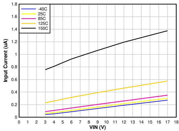
图 5-3. 典型关断电流
