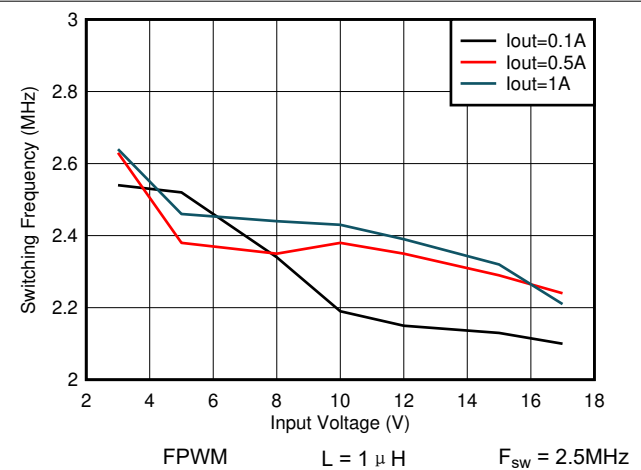
图 7-34. 开关频率与输入电压间的关系 V_{OUT} = 1.8V
