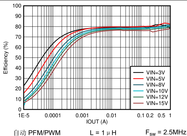
图 7-71. 效率与输出电流间的关系 V_{OUT} = 0.4V
