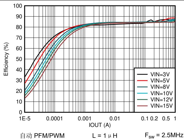
图 7-21. 效率与输出电流间的关系 V_{OUT} = 1.2V
