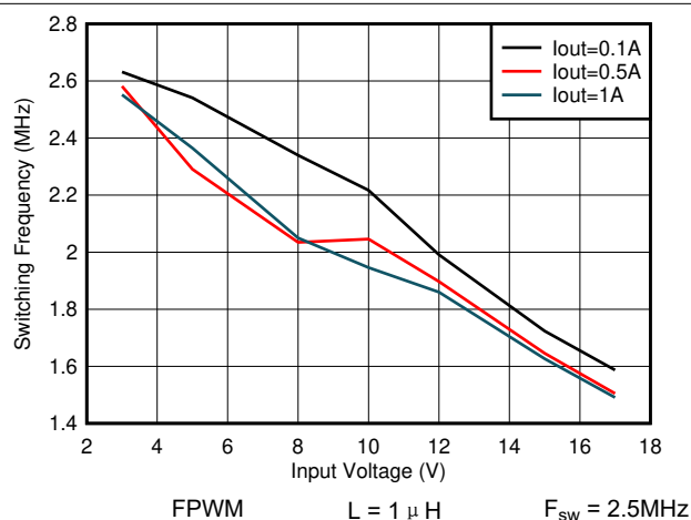
图 7-38. 开关频率与输入电压间的关系 V_{OUT} = 1.2V
