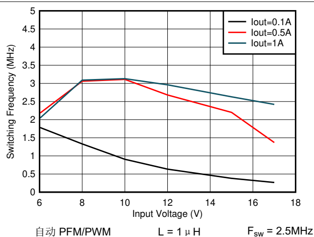
图 7-25. 开关频率与输入电压间的关系 V_{OUT} = 5V
