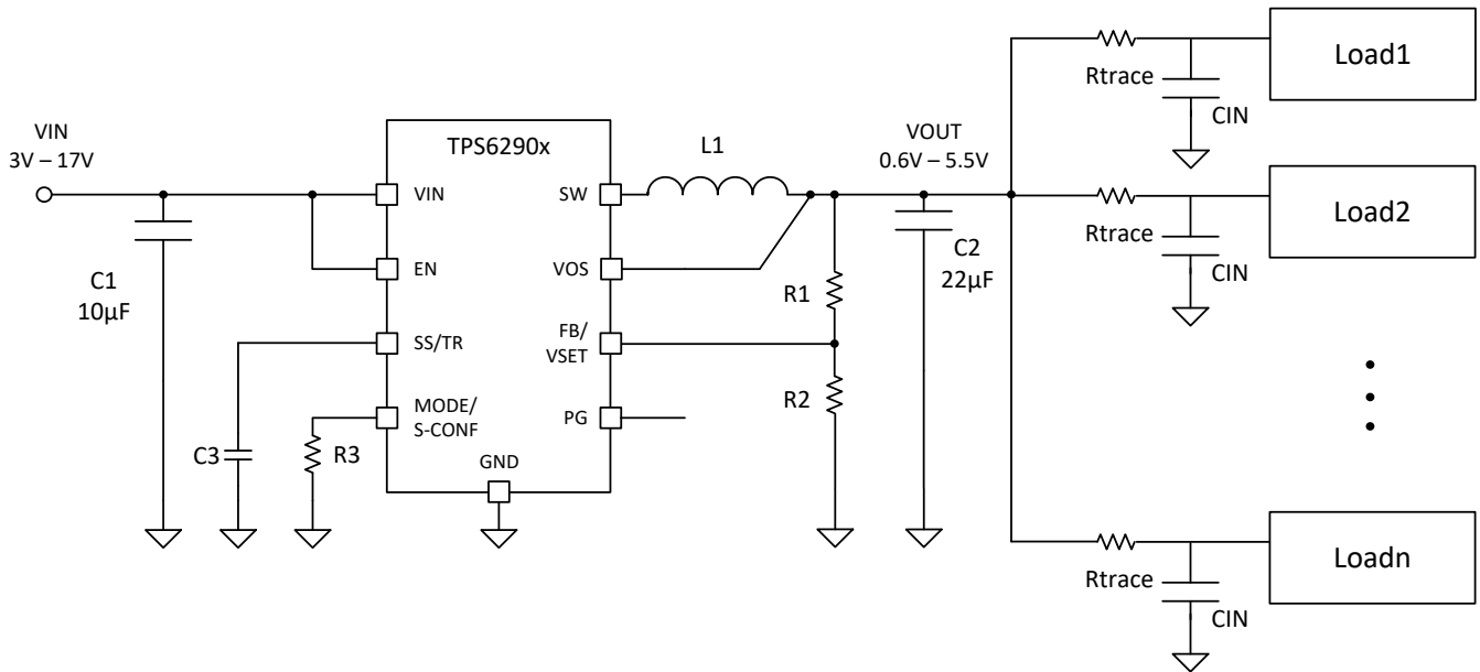
图 7-82. 多个负载
