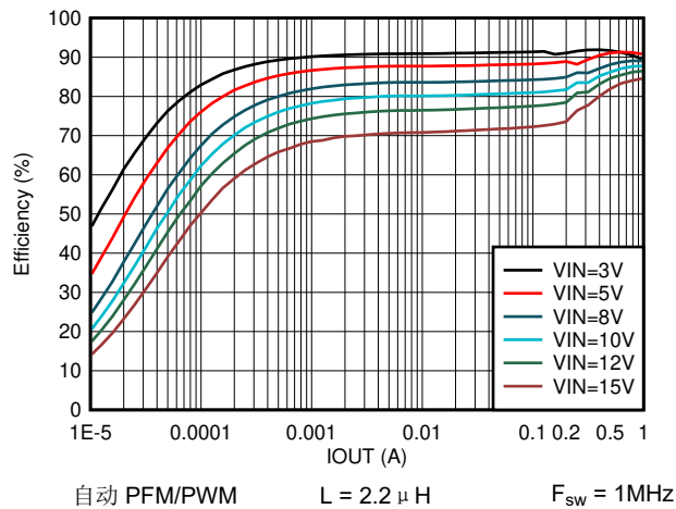
图 7-19. 效率与输出电流间的关系 V_{OUT} = 1.2V
