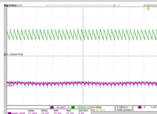
图 7-50. 输出电压纹波
