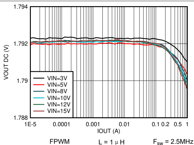
图 7-40. 输出电压与输出电流间的关系 V_{OUT} = 1.8V
