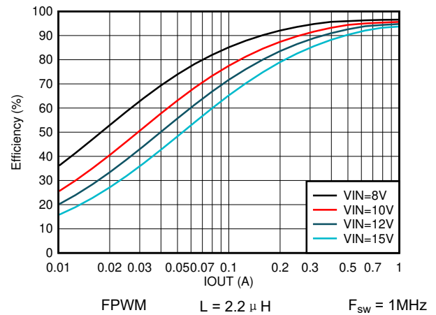
图 7-8. 效率与输出电流间的关系 V_{OUT} = 5V
