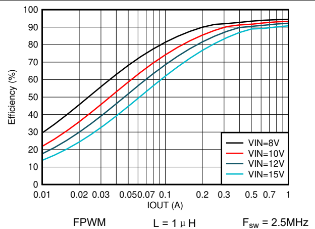
图 7-10. 效率与输出电流间的关系 V_{OUT} = 5V
