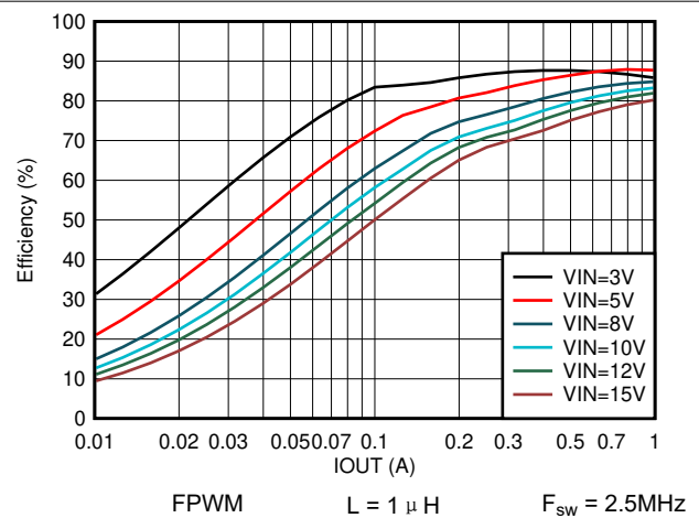
图 7-22. 效率与输出电流间的关系 V_{OUT} = 1.2V
