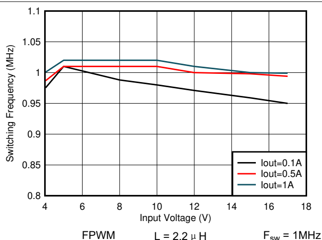
图 7-28. 开关频率与输入电压间的关系 V_{OUT} = 3.3V
