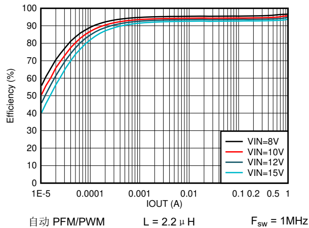
图 7-7. 效率与输出电流间的关系 V_{OUT} = 5V
