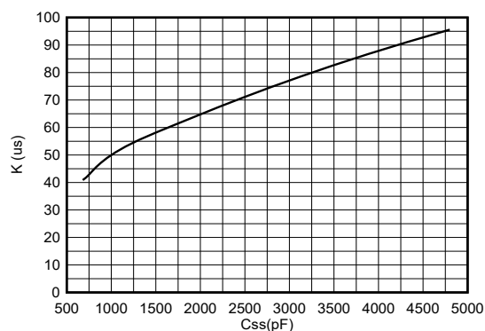
图 7-3. K 与 C_{SS} 关系曲线 (680pF-4800pF)
