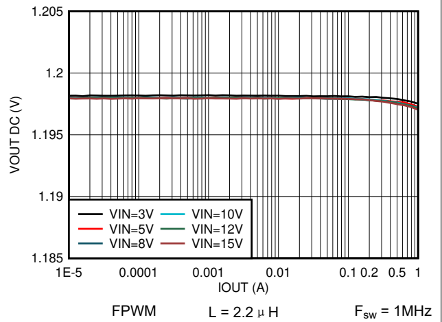
图 7-78. 输出电压与输出电流间的关系 V OUT = 1.2V
