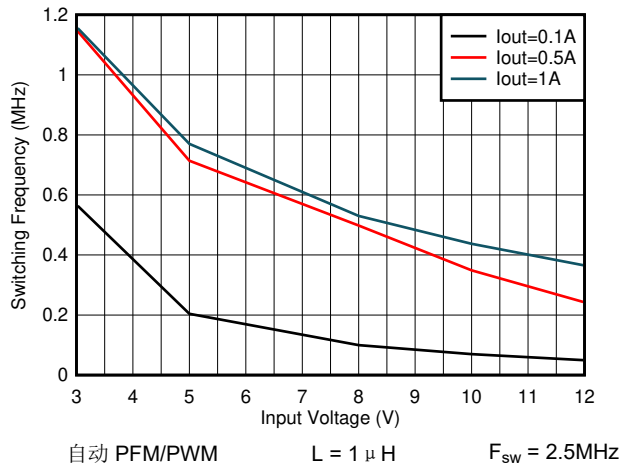
图 7-75. 开关频率与输入电压间的关系 V OUT = 0.4V
