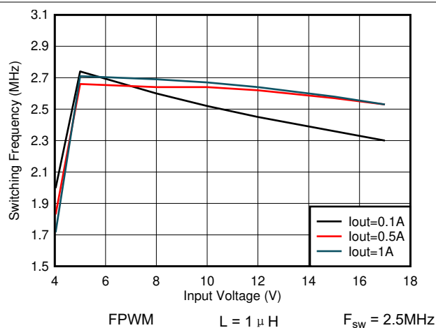
图 7-30. 开关频率与输入电压间的关系 V_{OUT} = 3.3V
