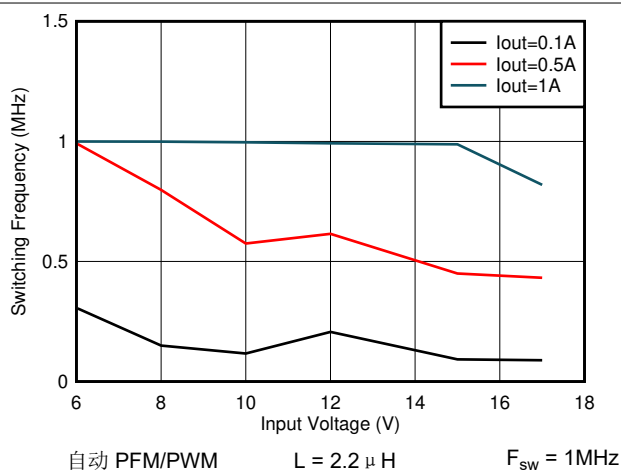
图 7-23. 开关频率与输入电压间的关系 V_{OUT} = 5V
