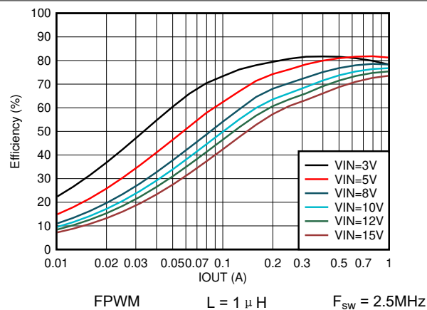
图 7-72. 效率与输出电流间的关系 V_{OUT} = 0.4V
