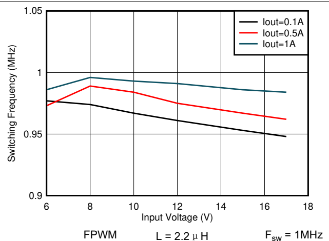
图 7-24. 开关频率与输入电压间的关系 V_{OUT} = 5V
