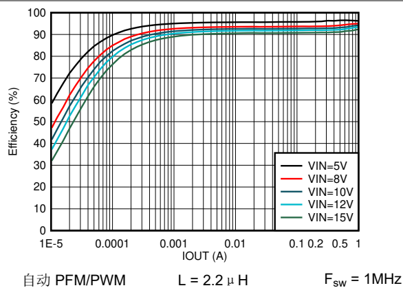
图 7-11. 效率与输出电流间的关系 V_{OUT} = 3.3V
