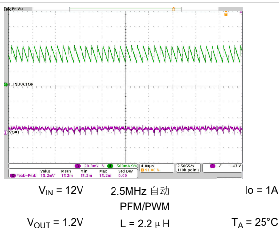
图 7-67. 输出电压纹波
