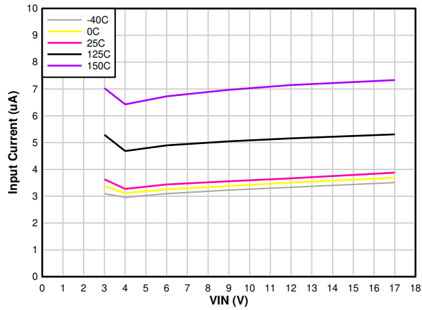
图 5-1. 典型静态电流与 V_{IN} 间的关系
