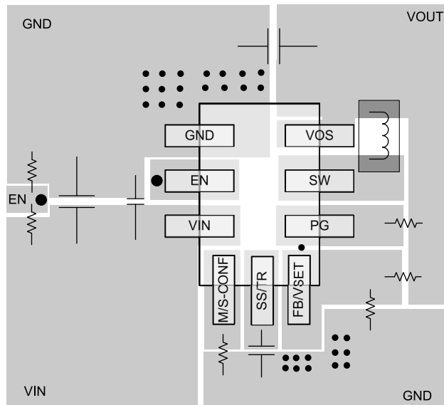
图 7-85. 布局
