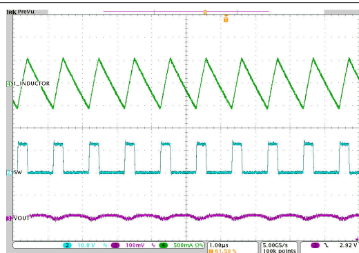
图 7-51. 输出电压纹波
