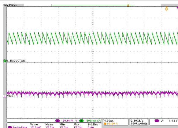
图 7-49. 输出电压纹波
