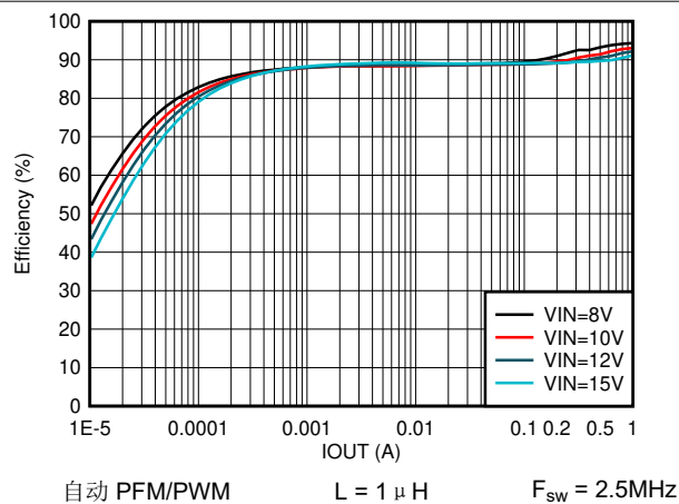
图 7-9. 效率与输出电流间的关系 V_{OUT} = 5V
