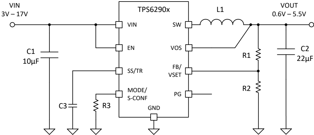
图 7-1. 典型应用电路
