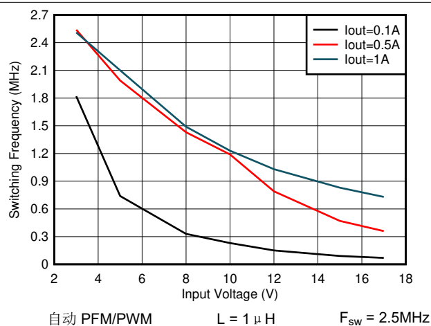
图 7-37. 开关频率与输入电压间的关系 V_{OUT} = 1.2V
