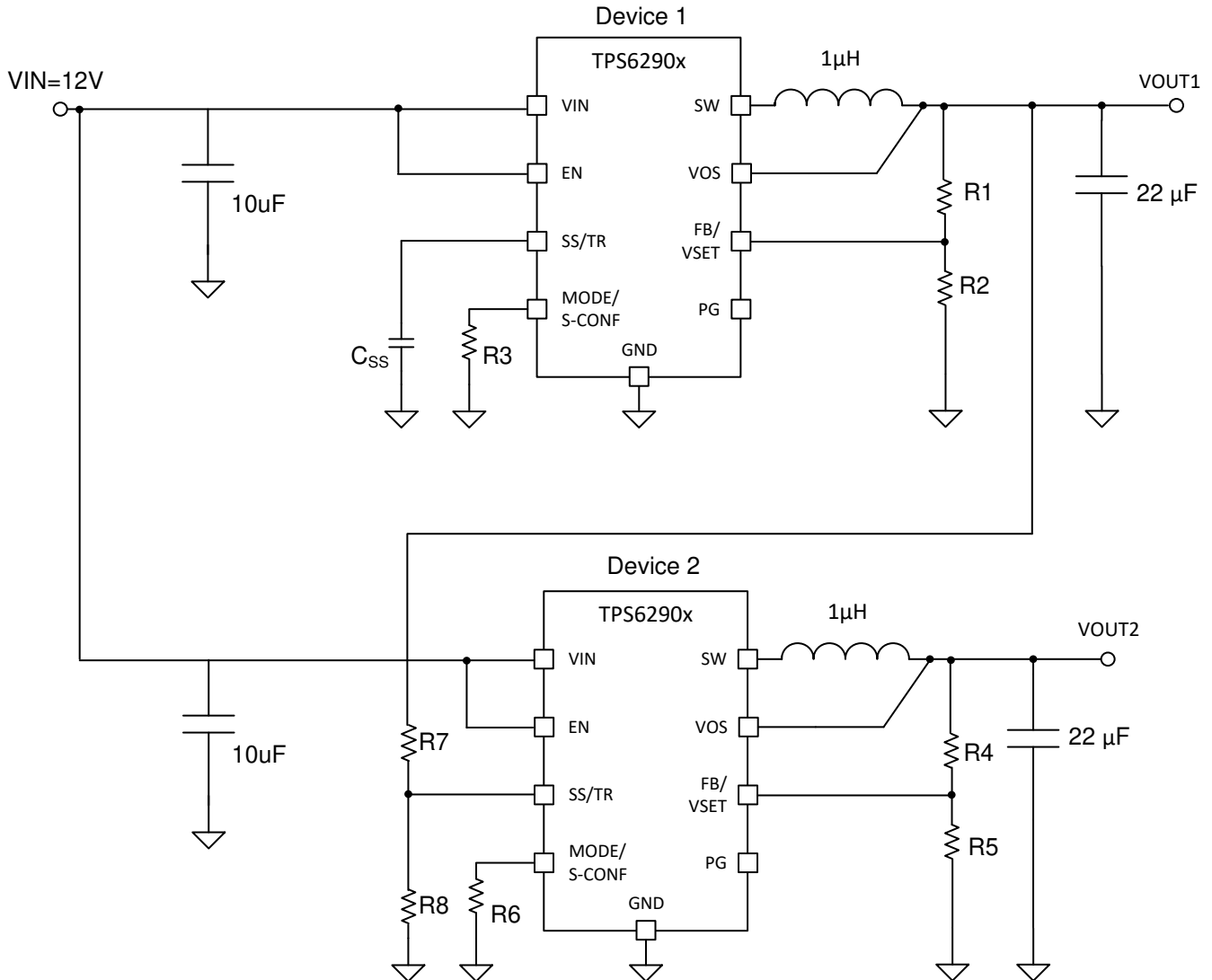
图 7-6. 比例式和同步启动原理图
