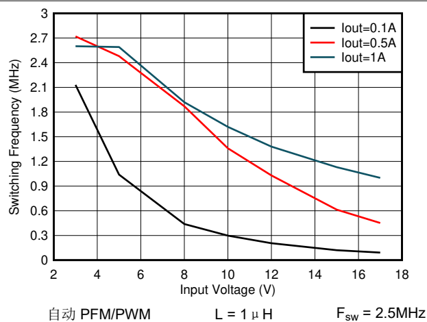
图 7-33. 开关频率与输入电压间的关系 V_{OUT} = 1.8V
