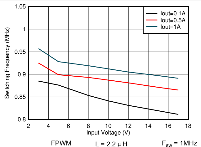
图 7-36. 开关频率与输入电压间的关系 V_{OUT} = 1.2V
