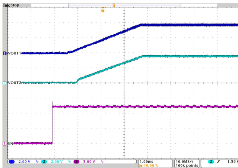
图 7-84. 跟踪
