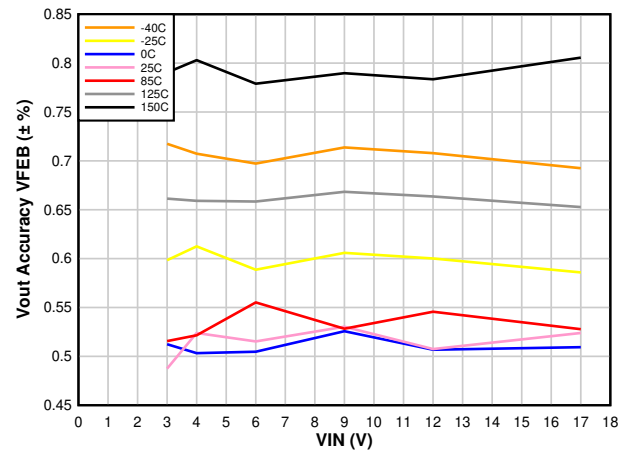
图 5-4. 输出电压精度 - 选择 VFEB
