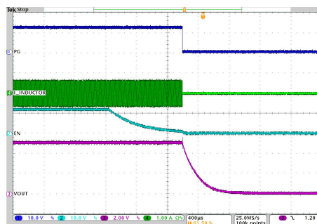
图 7-65. 输出放电功能 - 启用
