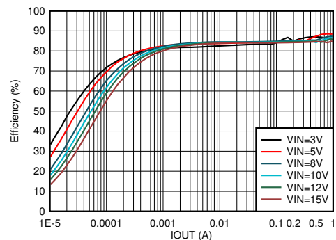
效率与输出电流间的关系 ( 1.2V O , 2.5MHz-1 \mu H, 自动 PFM/PWM )
