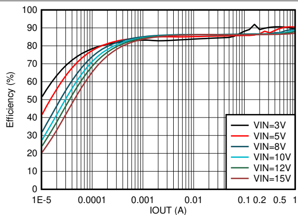
图 7-15. 效率与输出电流间的关系 V_{OUT} = 1.8V
