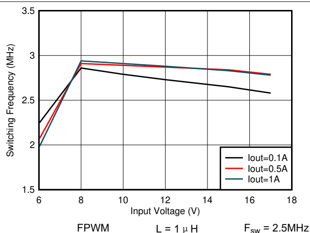
图 7-26. 开关频率与输入电压间的关系 V_{OUT} = 5V
