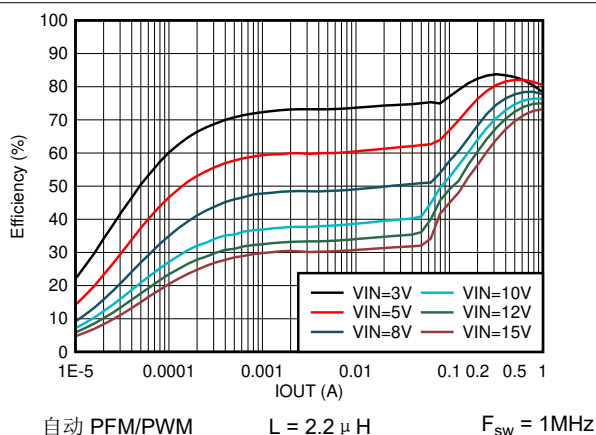
图 7-69. 效率与输出电流间的关系 V_{OUT} = 0.4V
