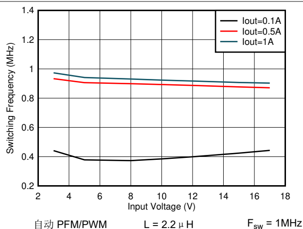
图 7-35. 开关频率与输入电压间的关系 V_{OUT} = 1.2V
