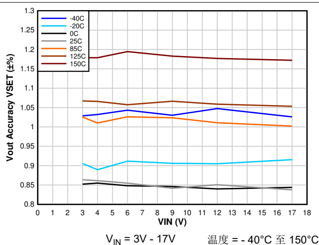
图 7-68. 输出电压精度 - 选择 VSET
