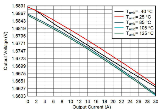
图 10-11. 输出电压与输出电流间的关系
