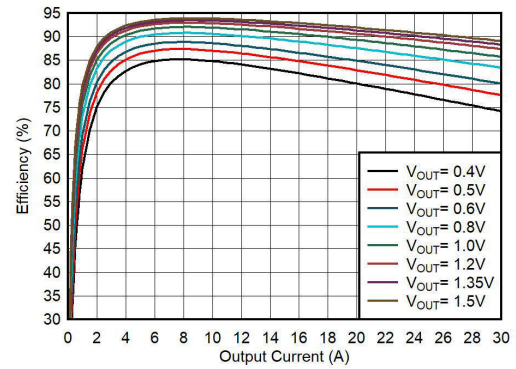
图 10-3. 效率与输出电流之间的关系
