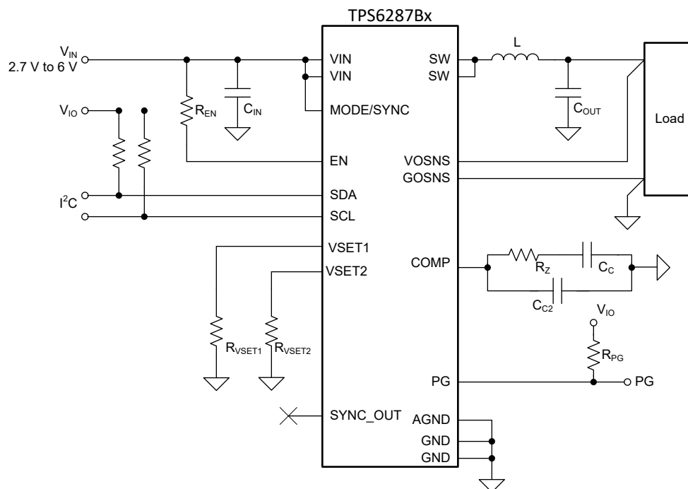
图 7-1. TPS6287Bx 的测量设置
