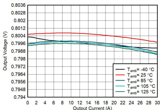
图 10-8. 输出电压与输出电流间的关系
