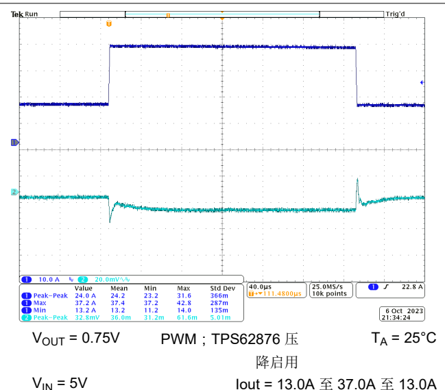
图 10-32. 负载瞬态响应
