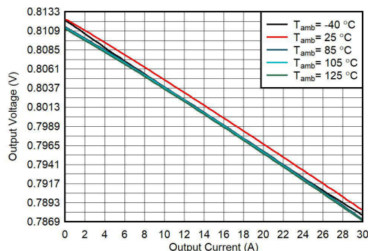
图 10-9. 输出电压与输出电流间的关系
