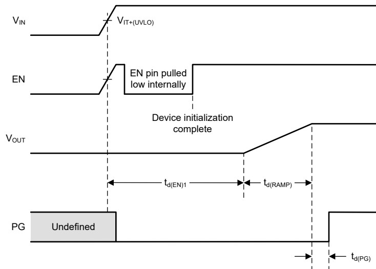
图 8-7. EN 上拉至 V_{\text{IN}} 时的启动时序
