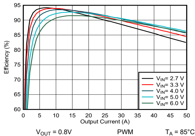
图 10-29. 效率与输出电流之间的关系
