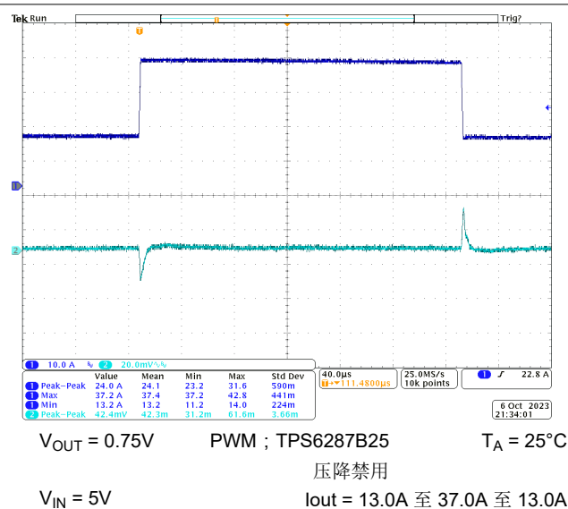
图 10-31. 负载瞬态响应
