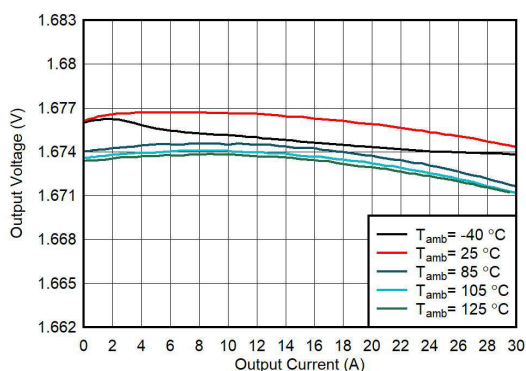
图 10-10. 输出电压与输出电流间的关系
