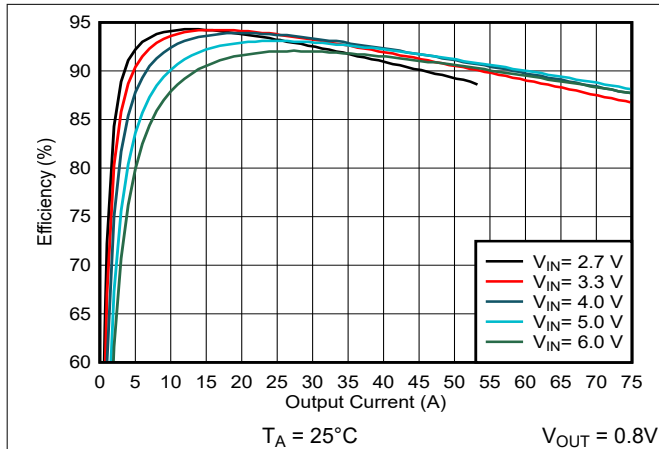
图 10-36. 效率与输出电流之间的关系
