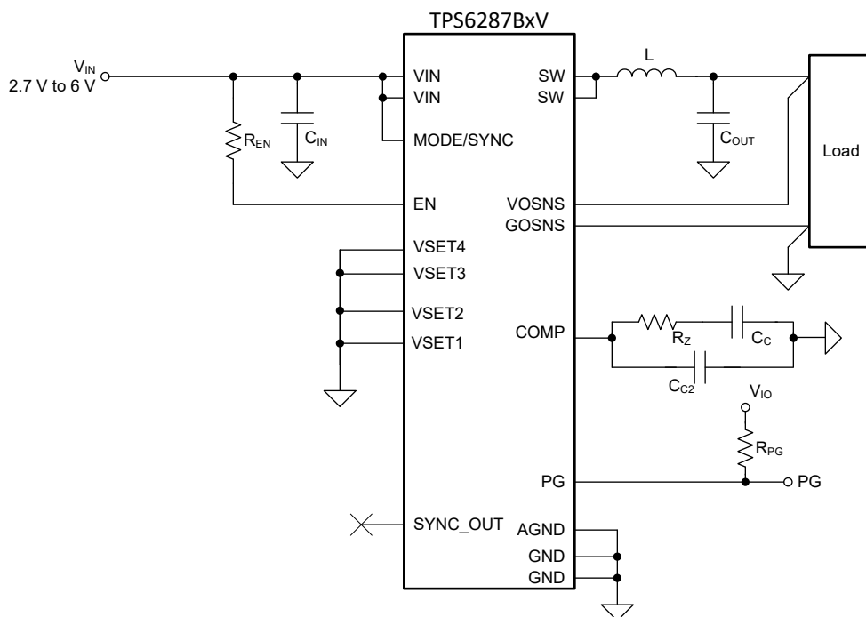
图 10-25. TPS6287BxV 的典型应用原理图
