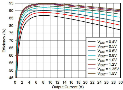
图 10-2. 效率与输出电流之间的关系
