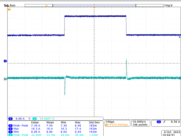
图 10-20. 启动时序
