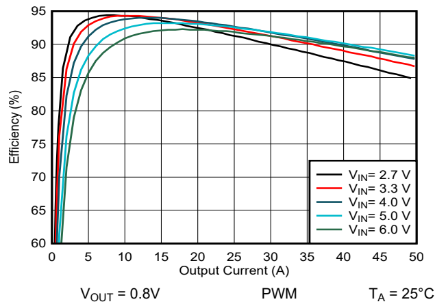
图 10-27. 效率与输出电流之间的关系
