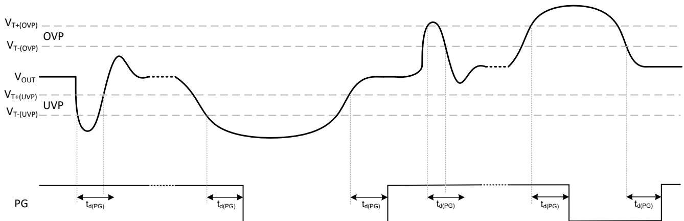
图 8-13. PG 时序
