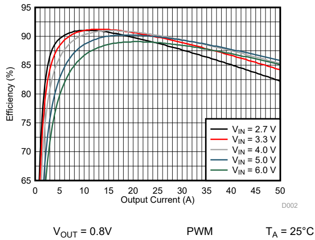
图 10-21. 效率与输出电流间的关系
