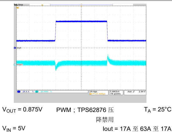
图 10-33. 负载瞬态响应
