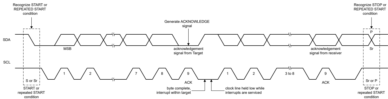
图 8-20. 总线协议
