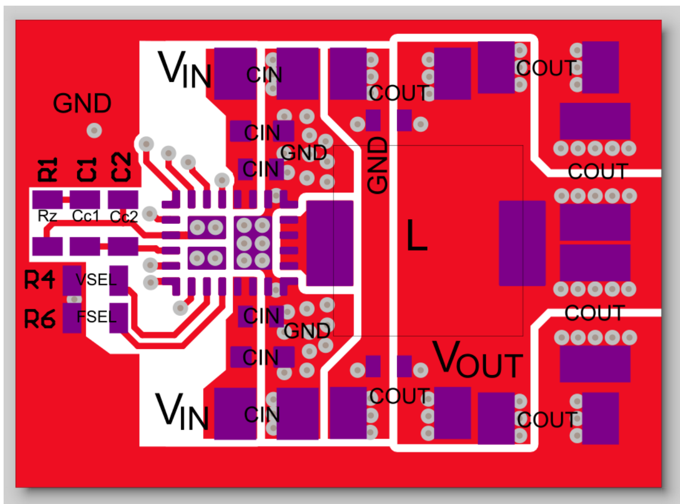
图 10-36. TPS62876-Q1 EVM 顶层
