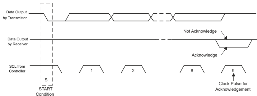
图 8-19. I²C 总线上的确认
