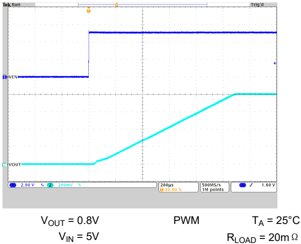
图 10-23. 启动时序
