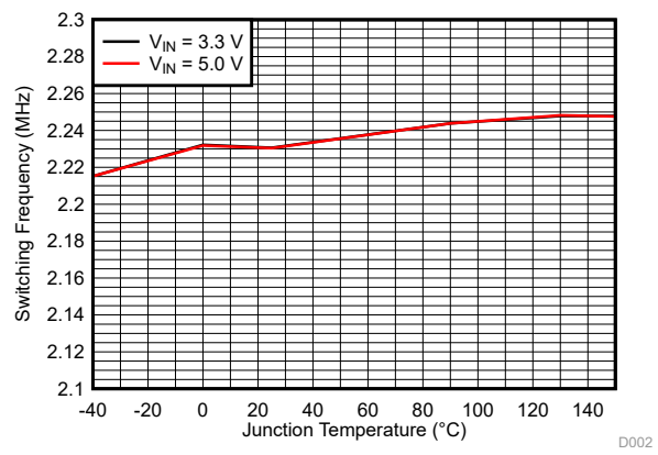
图 6-6. 开关频率与温度间的关系
