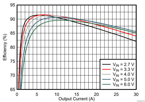
图 10-11. 效率与输出电流间的关系
