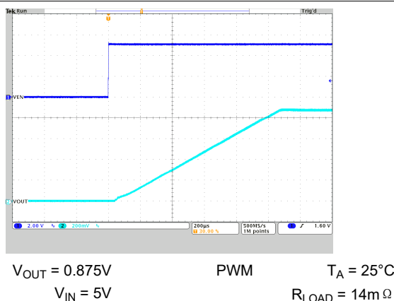
图 10-31. 启动时序
