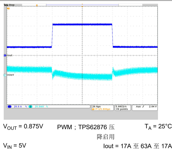
图 10-34. 负载瞬态响应
