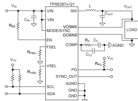
简化原理图
