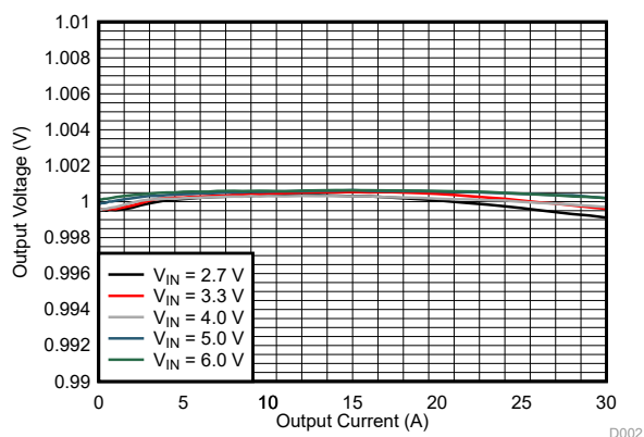
图 10-10. 输出电压与输出电流间的关系
