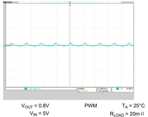
图 10-24. 输出电压纹波
