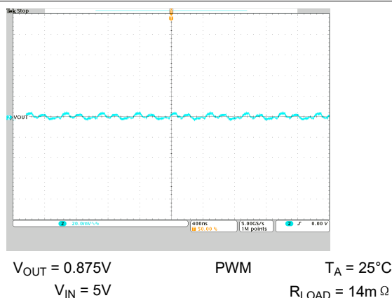
图 10-32. 输出电压纹波
