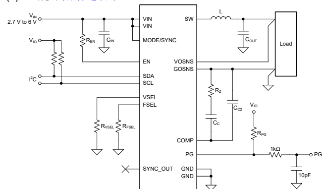
TPS6287x 简化原理图
