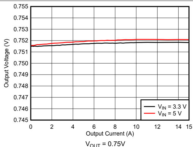
图 10-7. 负载调整率
