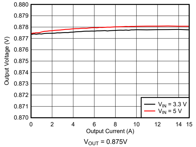
图 10-9. 负载调整率
