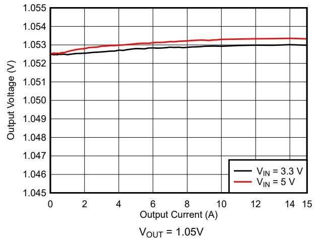
图 10-11. 负载调整率
