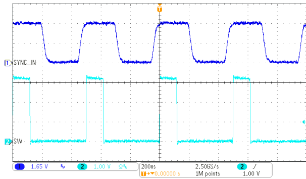
图 10-20. 可与外部时钟保持同步
