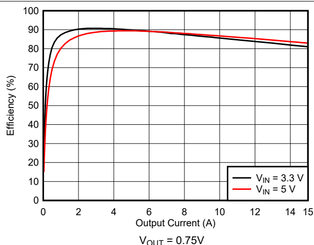
图 10-6. 效率
