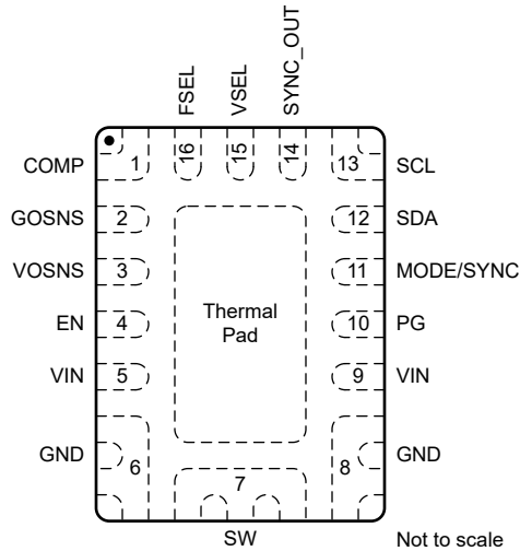
图 6-1. 16 引脚 RXS VQFN 封装 (顶视图)
