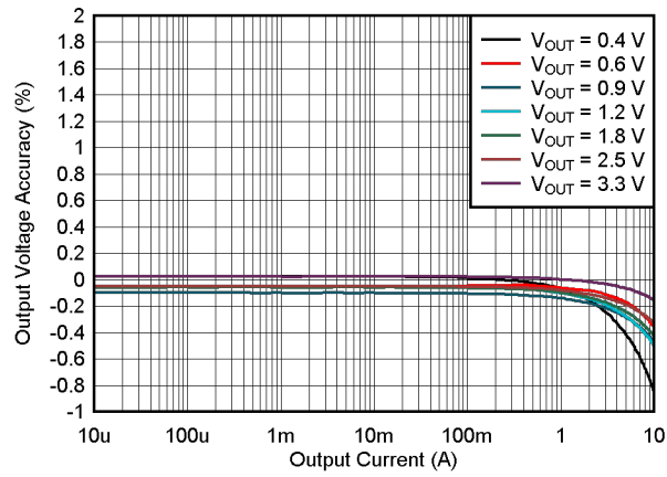
图 9-10. 负载调整率
