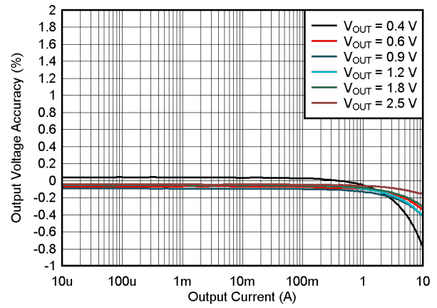
图 9-11. 负载调整率
