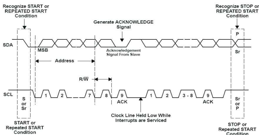
图 7-9. 总线协议
