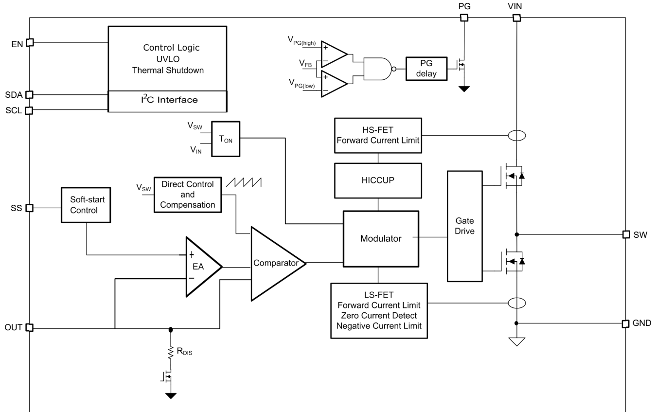
图 7-2. 功能方框图 - I²C 版本 (TPS6286Bxx)
