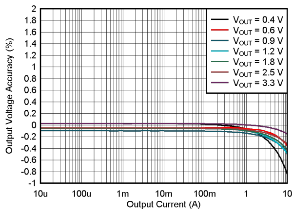
图 9-10. 负载调整率
