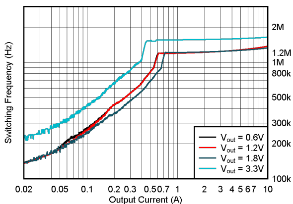
图 9-15. 开关频率
