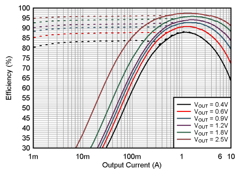
图 9-5. 效率与输出电流之间的关系
