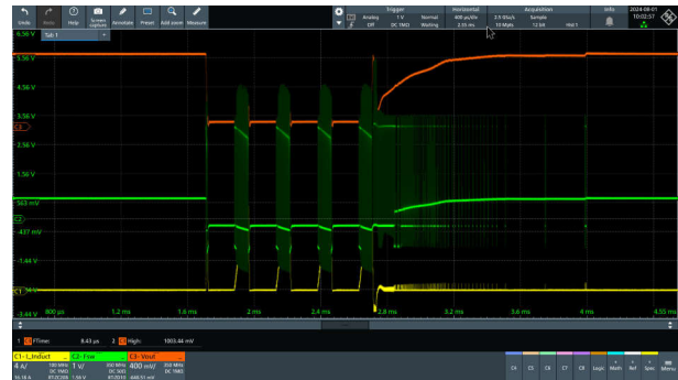
图 9-35. 断续短路保护
