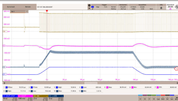
图 9-27. 负载瞬态 - FPWM 运行
