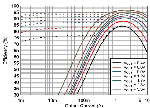
图 9-4. 效率与输出电流之间的关系
