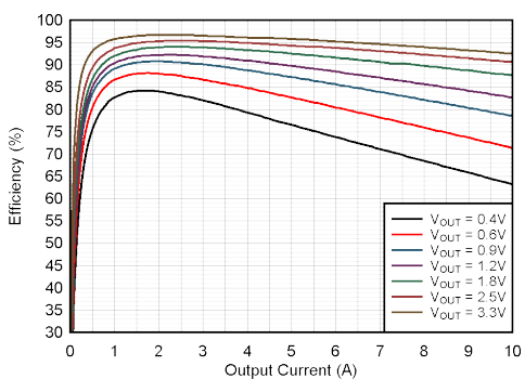
图 9-6. 效率与输出电流之间的关系
