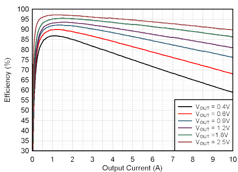
图 9-7. 效率与输出电流之间的关系
