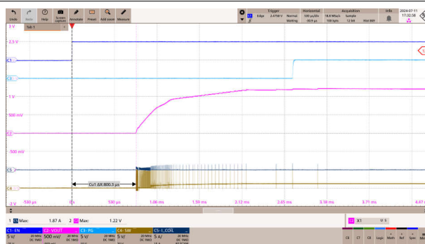
图 9-21. FPWM 运行
