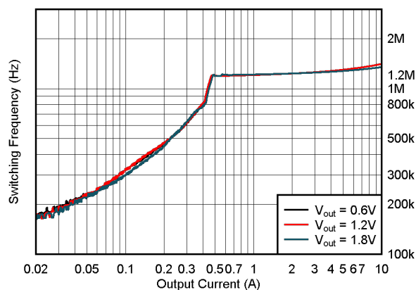
图 9-14. 开关频率
