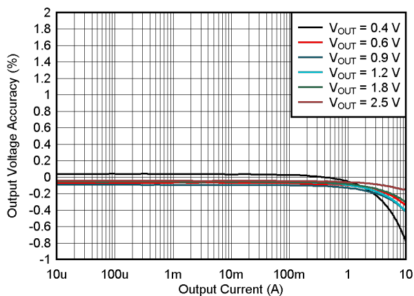
图 9-11. 负载调整率
