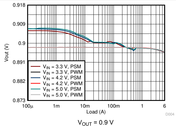
图 9-5. Load Regulation
