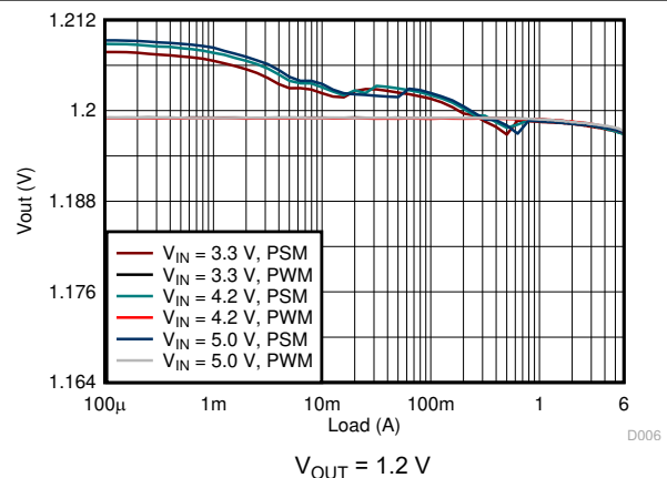
图 9-7. Load Regulation
