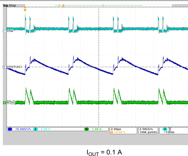
图 9-13. PSM Operation
