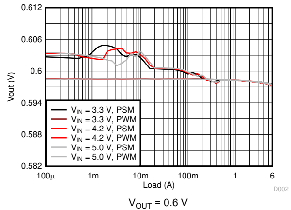
图 9-3. Load Regulation
