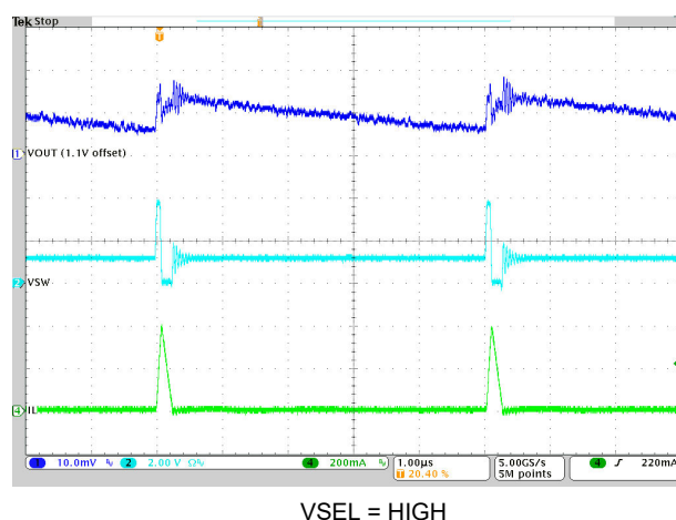
图 9-10. PFM Mode Operation
