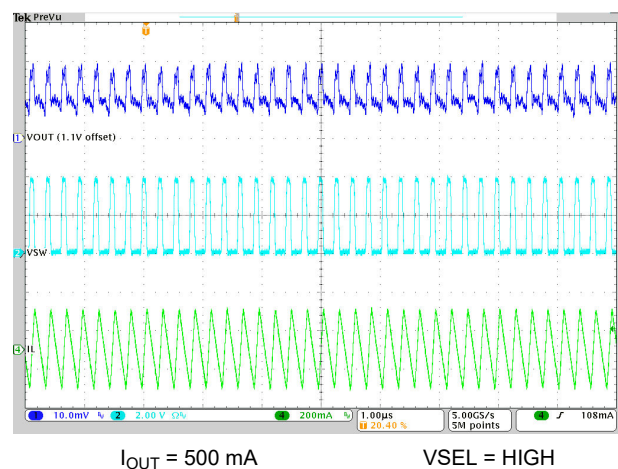
图 9-11. PWM-Mode Operation
