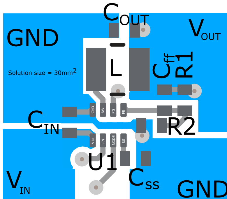
图 12-1. Example Layout
