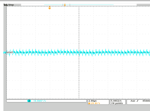
图 9-47. 输出电压纹波
