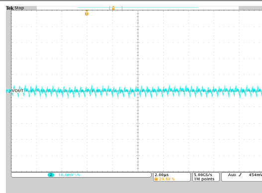
图 9-45. 输出电压纹波
