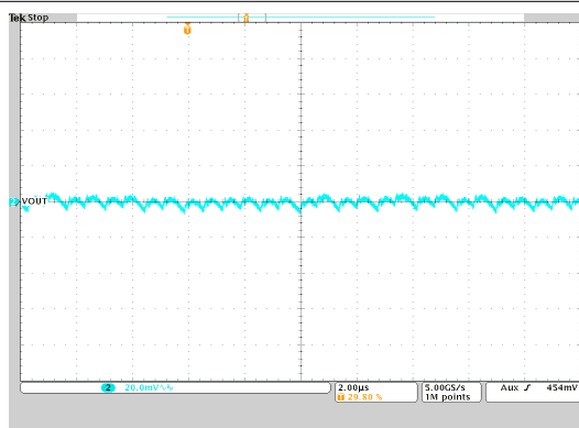
图 9-44. 输出电压纹波
