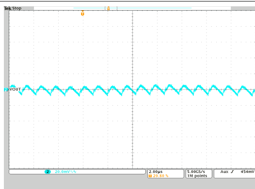
图 9-46. 输出电压纹波
