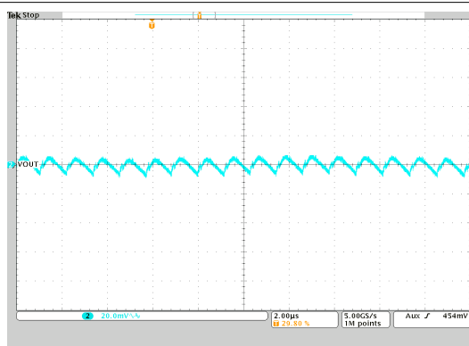
图 9-46. 输出电压纹波
