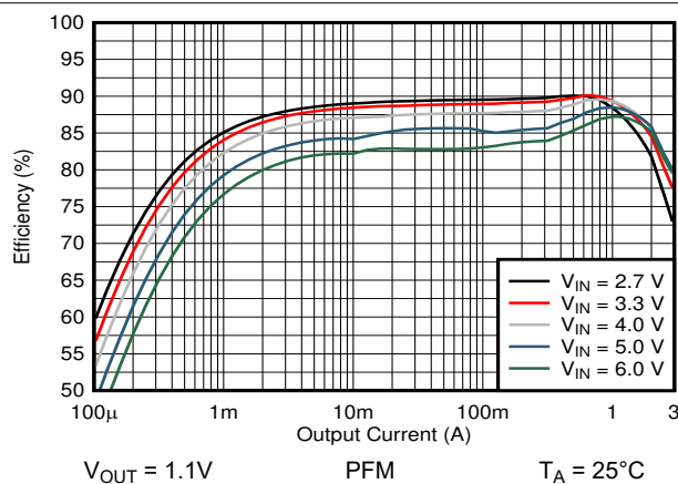
图 9-6. 效率与输出电流间的关系
