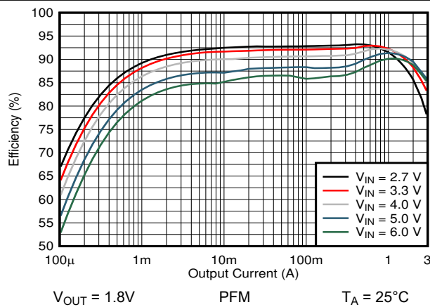
图 9-4. 效率与输出电流间的关系
