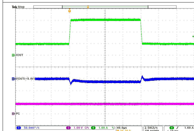
图 8-33. Load Transient
