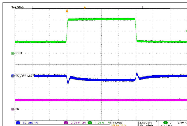
图 8-33. Load Transient
