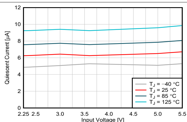
图 6-4. Quiescent Current
