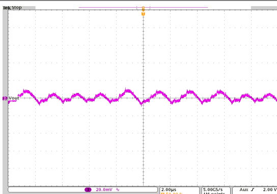
图 9-44. 输出电压纹波
