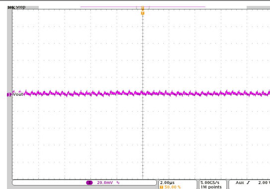
图 9-45. 输出电压纹波
