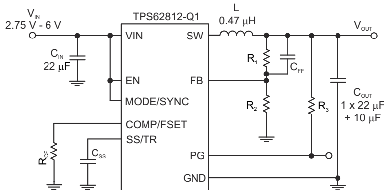
图 7-2. TPS62812-Q1 和 TPS62811-Q1 的测量设置
