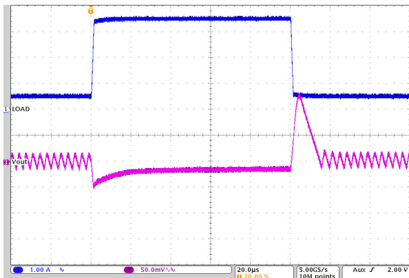
图 10-28. Load Transient Response
