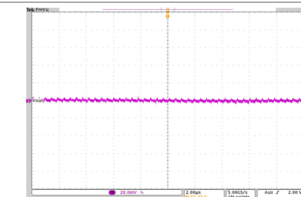
图 10-47. Output Voltage Ripple
