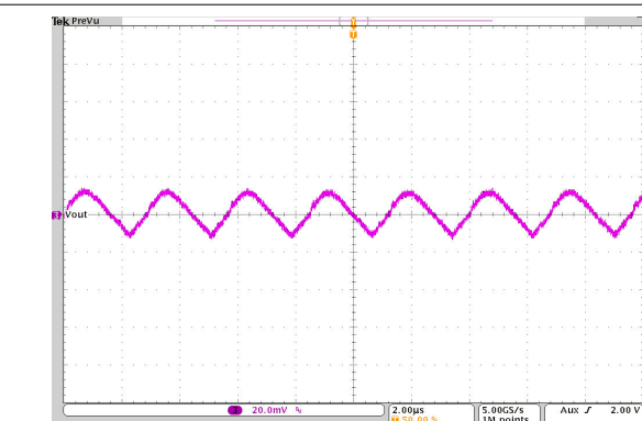
图 10-46. Output Voltage Ripple
