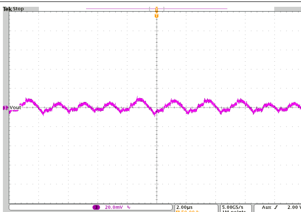
图 10-44. Output Voltage Ripple
