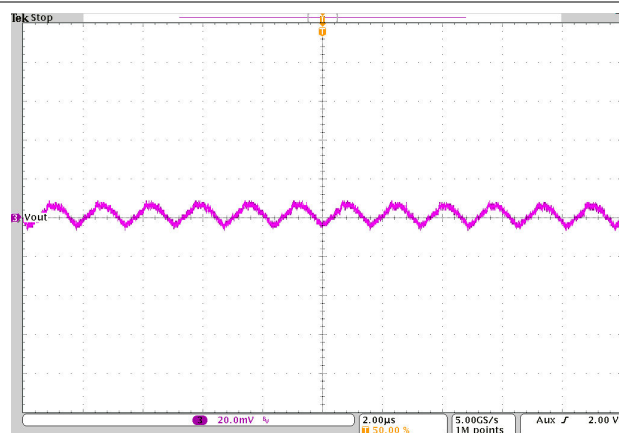
图 9-44. 输出电压纹波
