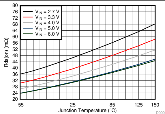
图 6-1. 高侧开关的 R_{ds(on)}
