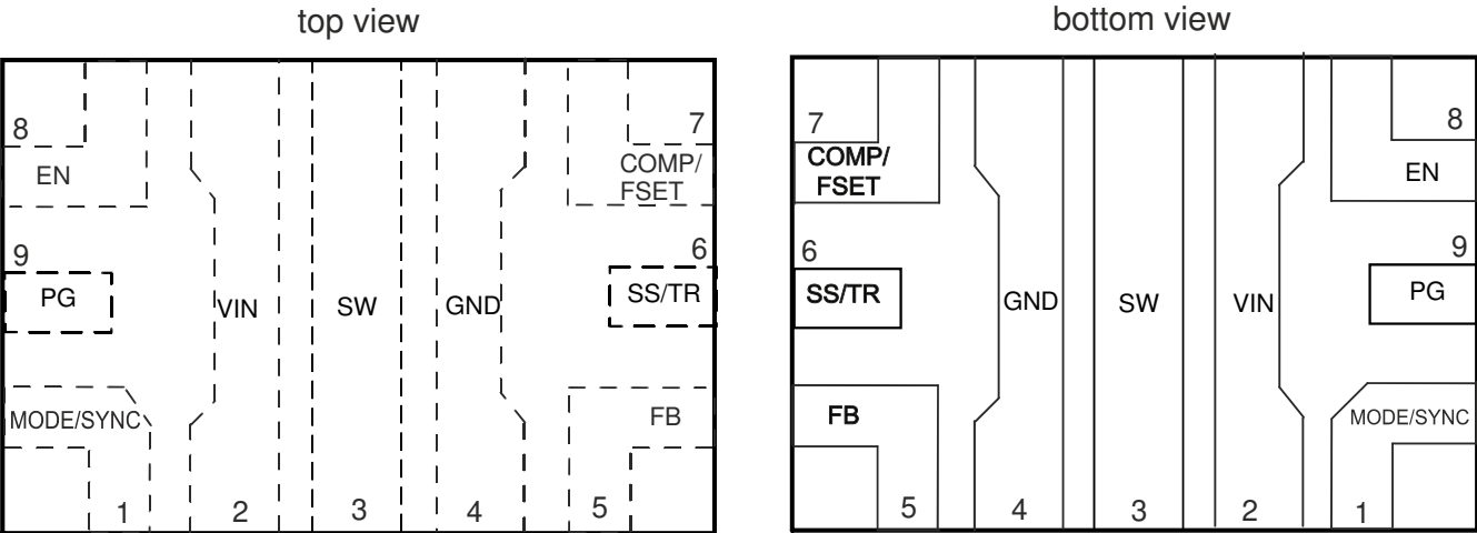
图 5-1.9 引脚 (VQFN-HR) RWY 封装
