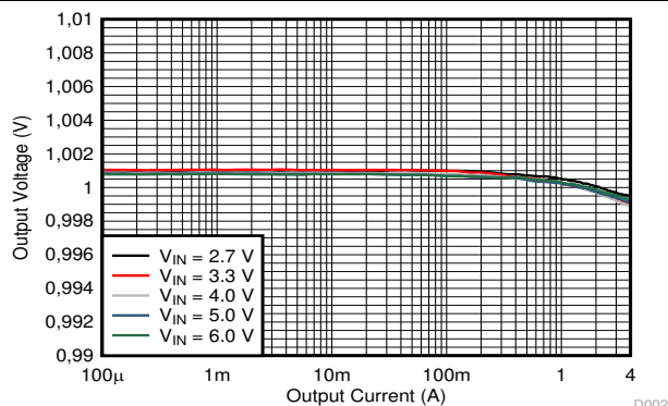
图 9-17. 输出电压与输出电流间的关系
