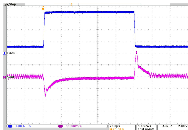
图 9-26. 负载瞬态响应
