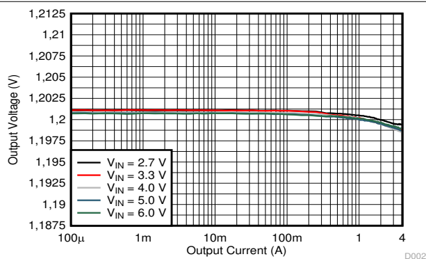
图 9-15. 输出电压与输出电流间的关系
