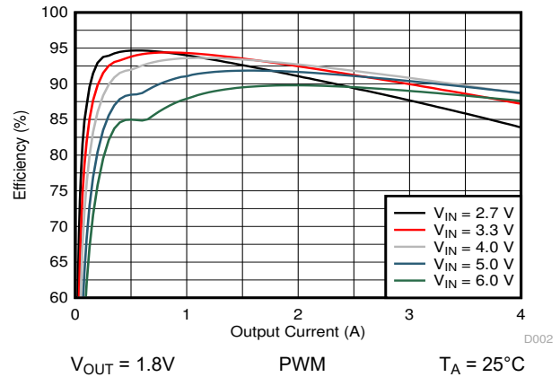
图 9-5. 效率与输出电流间的关系
