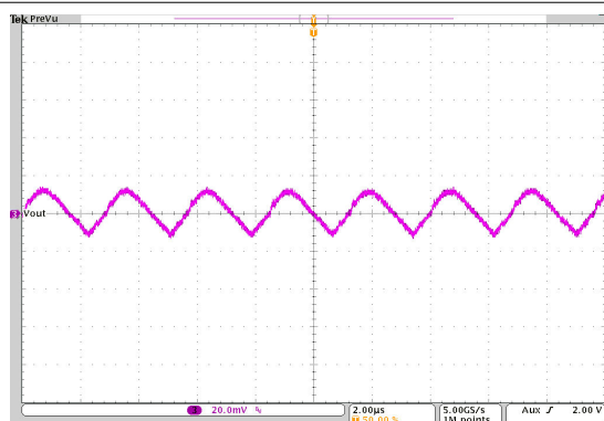
图 9-46. 输出电压纹波
