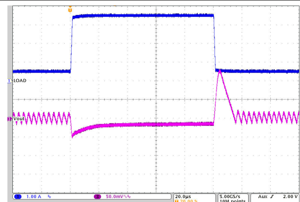
图 9-28. 负载瞬态响应
