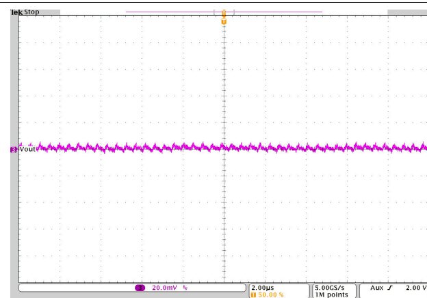
图 9-45. 输出电压纹波
