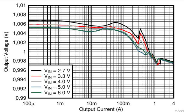
图 9-16. 输出电压与输出电流间的关系
