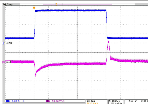
图 9-27. 负载瞬态响应
