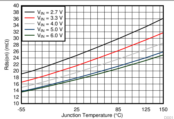
图 6-2. 低侧开关的 R_{ds(on)}
