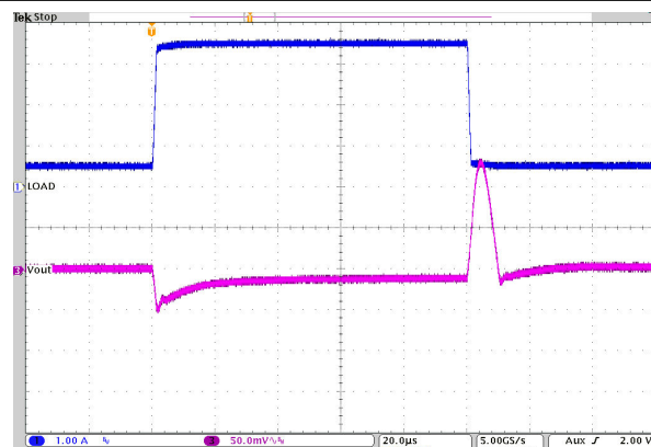
图 9-29. 负载瞬态响应
