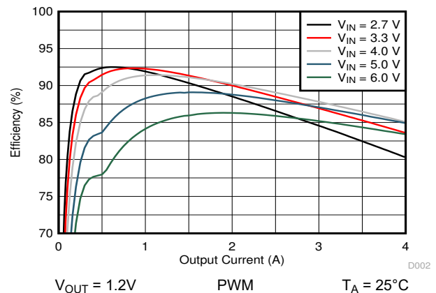
图 9-7. 效率与输出电流间的关系
