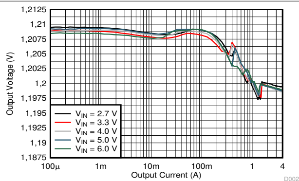
图 9-14. 输出电压与输出电流间的关系
