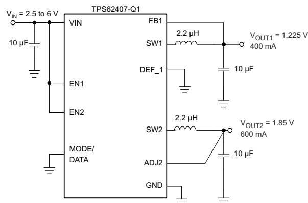
图 9-22. TPS62407-Q1 Fixed 1.225-V and 1.85-V Outputs
