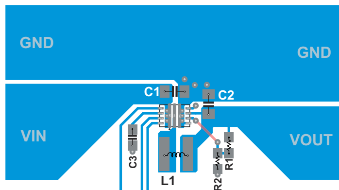
图 10-85. Layout
