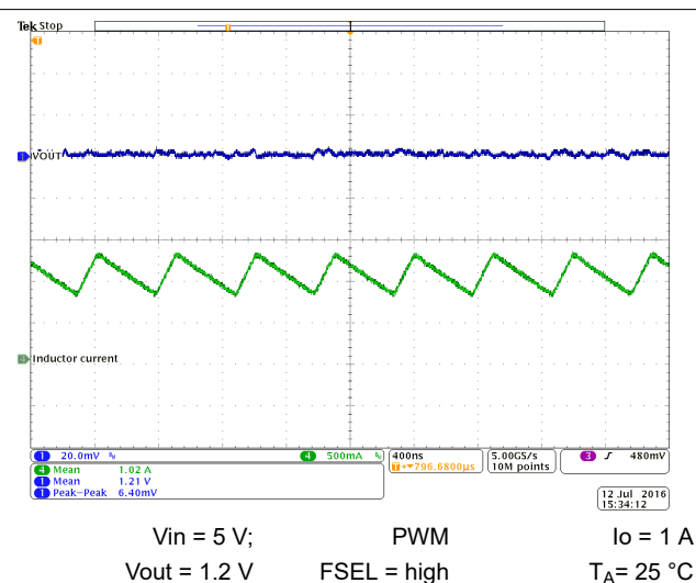
图 10-37. Output Voltage Ripple
