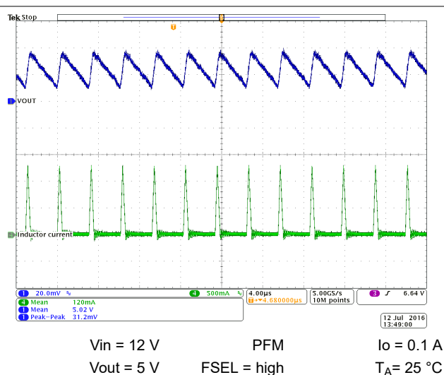
图 10-57. Output Voltage Ripple
