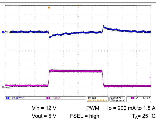
图 10-53. Load Transient Response
