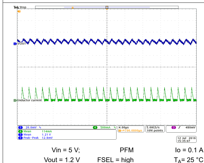
图 10-36. Output Voltage Ripple
