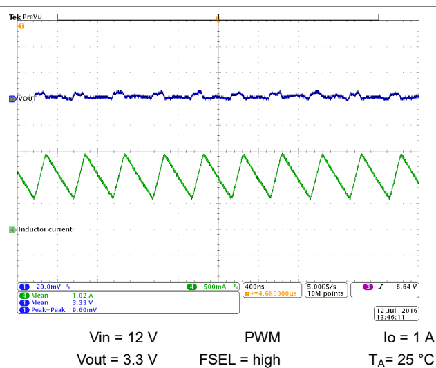
图 10-51. Output Voltage Ripple
