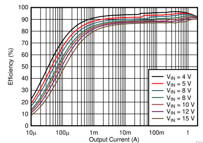
效率与输出电流间的关系， V_o = 3.3V ； f_{sw} = 1.25MHz ；PFM
