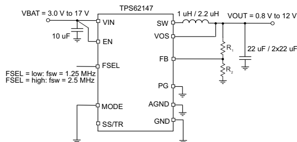
简化原理图
