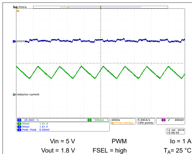
图 10-44. Output Voltage Ripple
