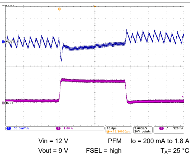
图 10-59. Load Transient Response
