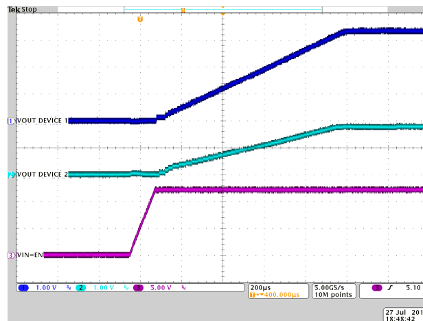
图 10-86. Tracking
