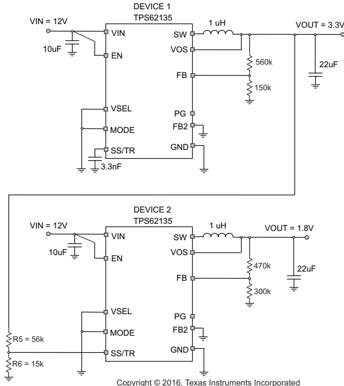
图 10-85. Tracking Example
