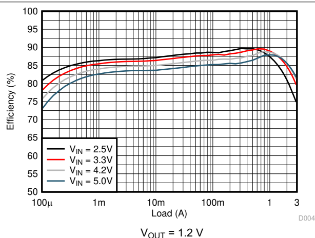
图 8-11. Efficiency
