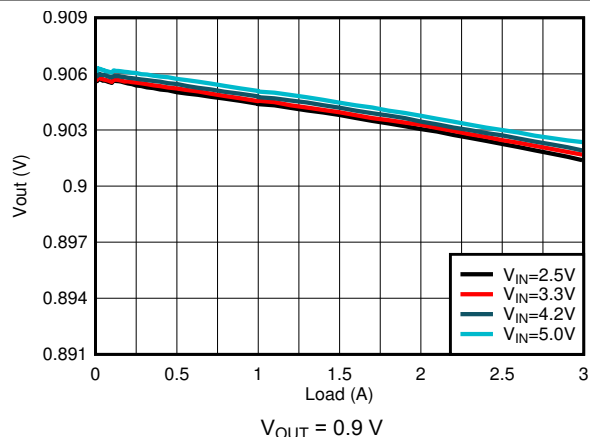
图 8-10. Load Regulation
