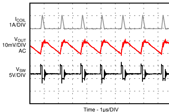
图 8-28. PSM Operation
