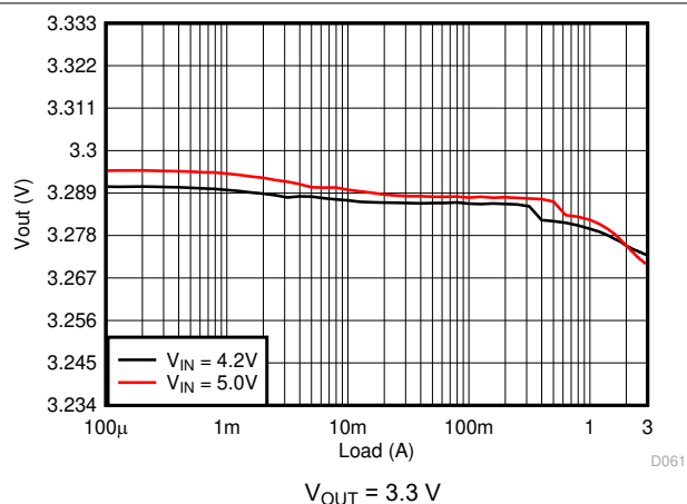
图 8-20. Load Regulation
