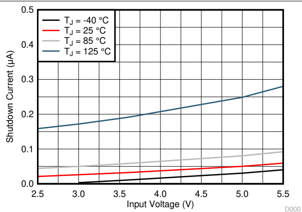
图 6-4. Shutdown Current
