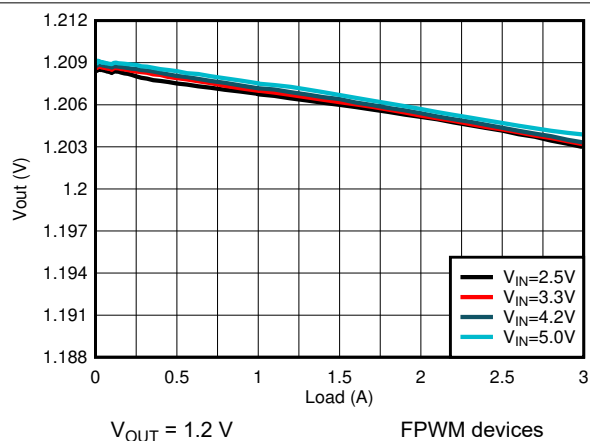
图 8-14. Load Regulation
