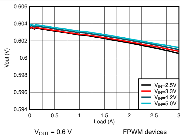
图 8-6. Load Regulation
