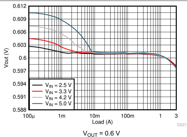
图 8-4. Load Regulation
