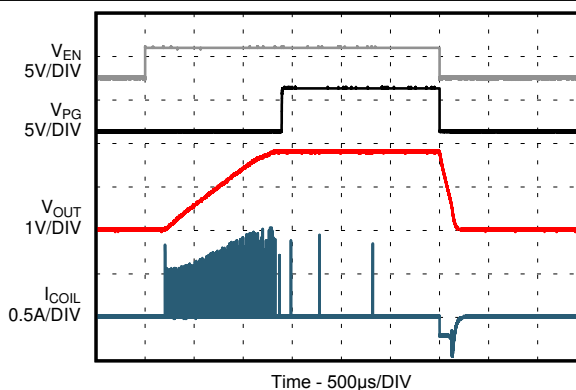
图 8-28. PSM Operation
