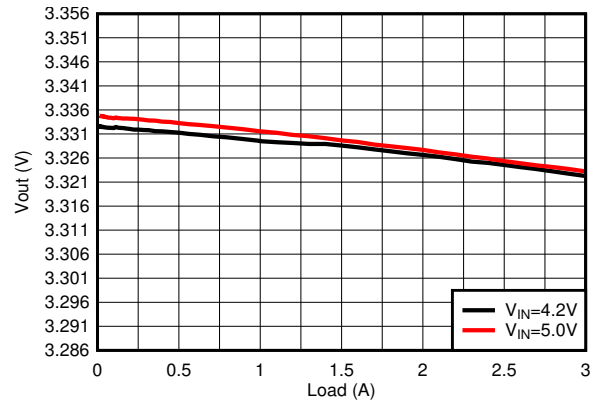
图 8-22. Load Regulation
