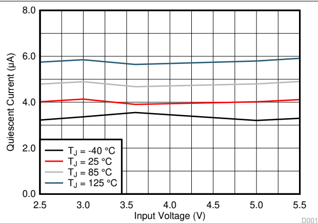
图 6-3. Quiescent Current
