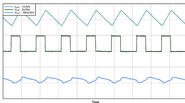
图 8-27. PWM Operation
