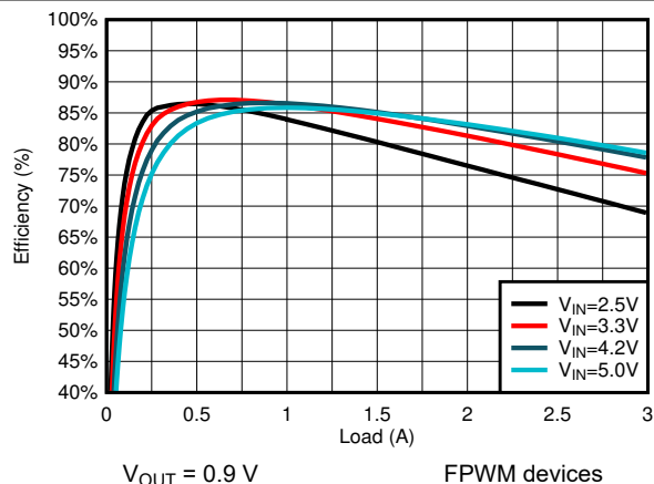
图 8-9. Efficiency
