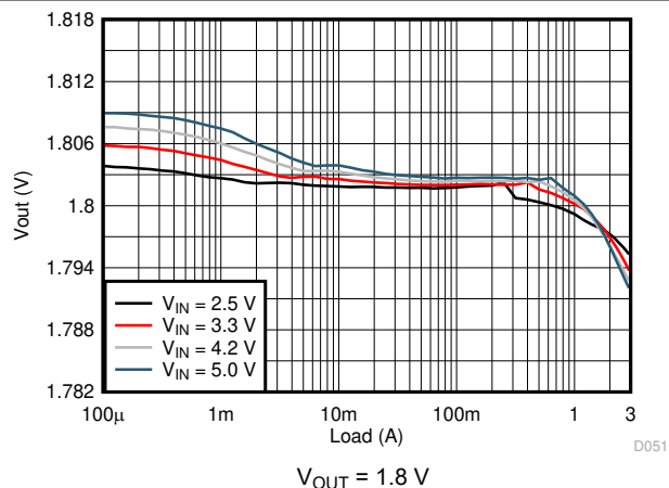
图 8-16. Load Regulation
