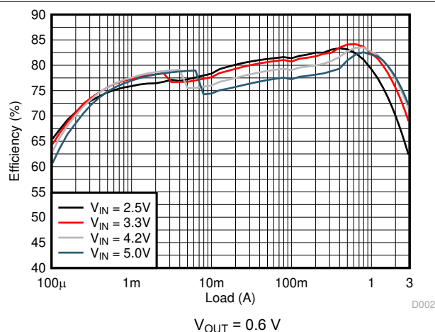
图 8-3. Efficiency
