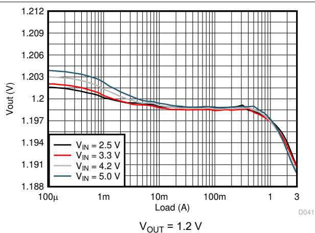
图 8-12. Load Regulation
