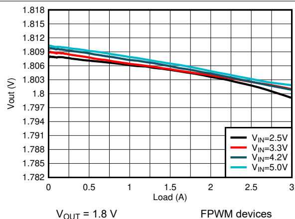
图 8-18. Load Regulation
