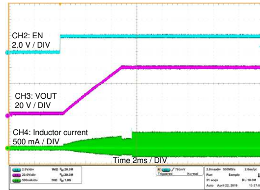
图 17. Startup
