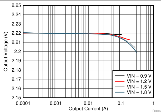
图 6-2. Load Regulation
