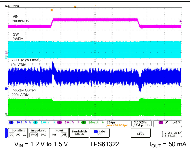
图 8-5. Line Transient
