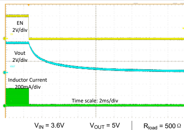
图 8-7. 由 EN 关断
