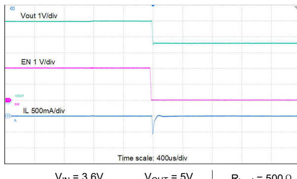
图 8-25. 由 EN 关断
