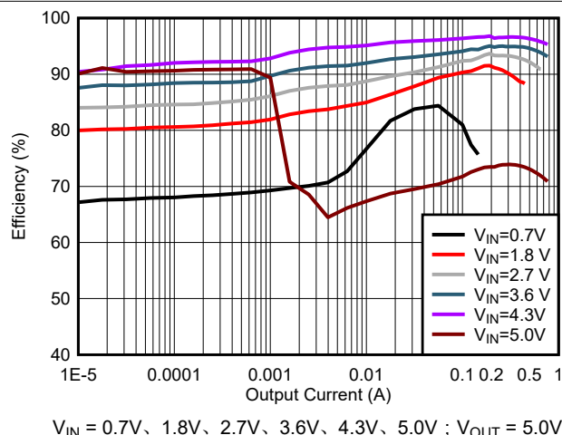
图 6-1. 不同输入电压在正常模式下的 5.0V VOUT 效率
