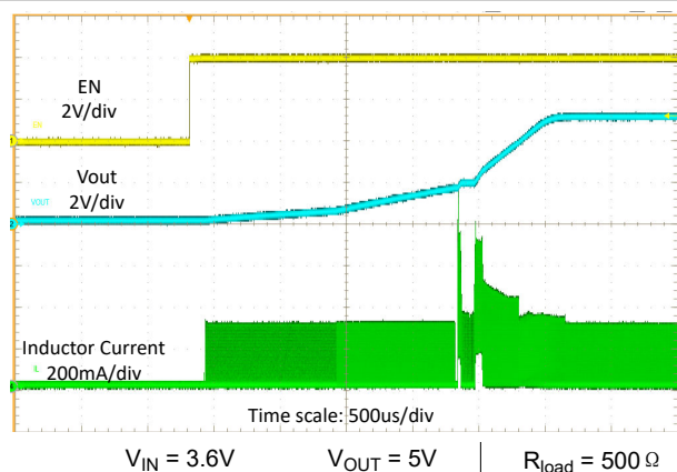
图 8-6. 由 EN 启动
