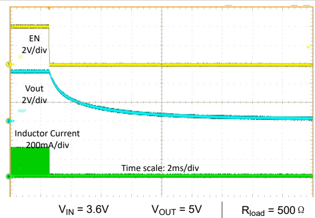
图 8-18. 由 EN 关断
