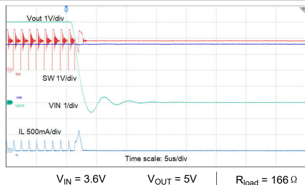
图 8-26. 短路保护
