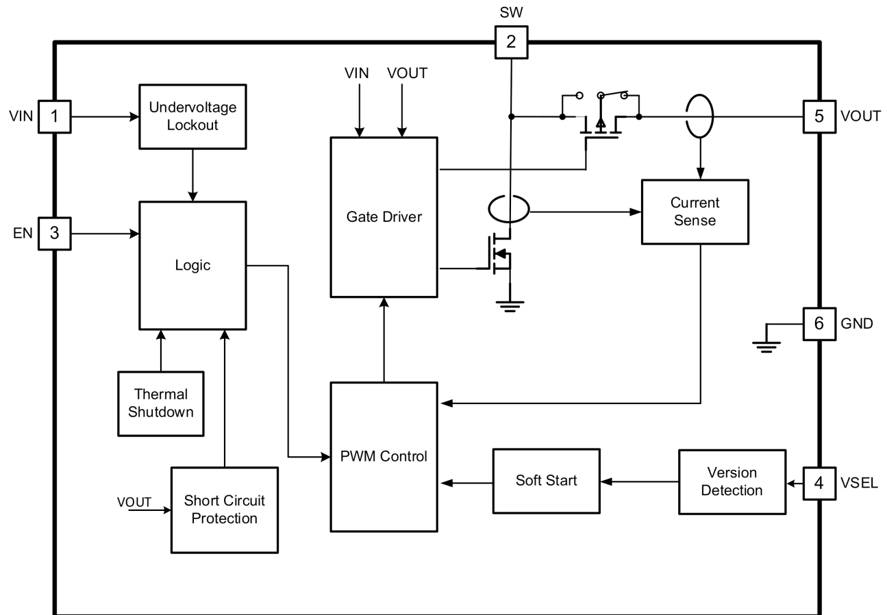
图 7-1. 功能方框图
