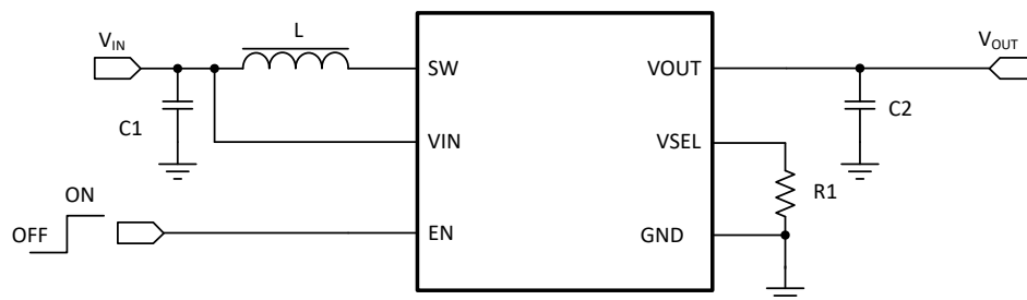
典型应用
