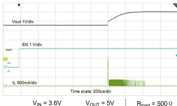
图 8-24. 由 EN 启动
