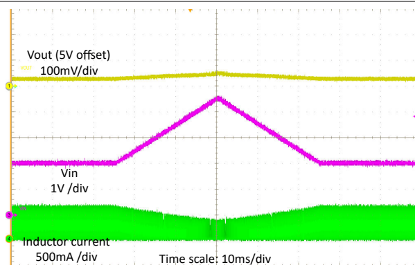
图 8-22. 线路扫描
