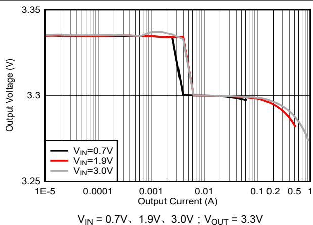
图 6-4. 正常模式下的 3.3V VOUT 负载调整率
