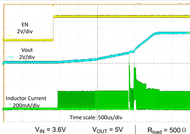
图 8-17. 由 EN 启动
