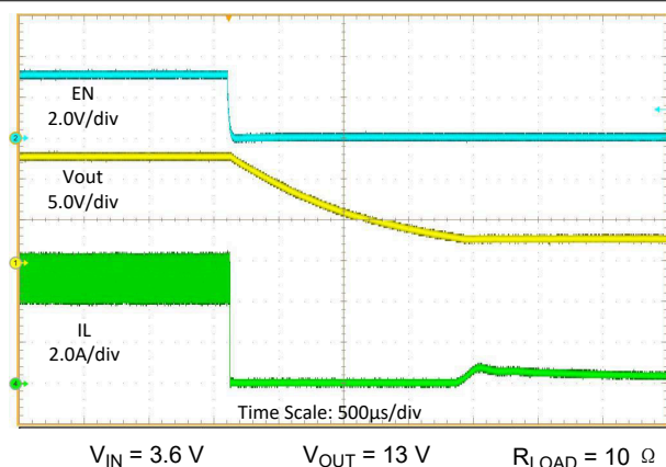
图 9-6. Shutdown Waveforms
