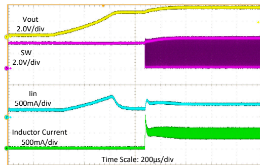
图 8-11. Line Sweep
