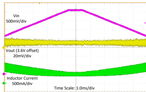
图 8-9. Line Transient
