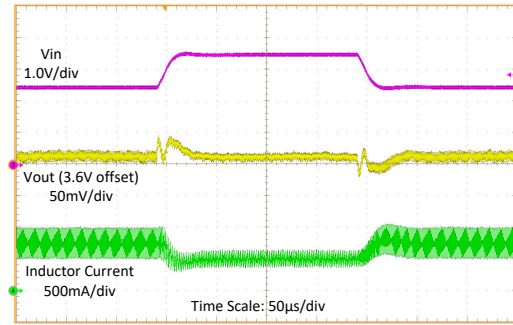
图 8-9. Line Transient
