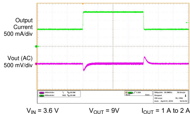
图 9-7. Load Transient
