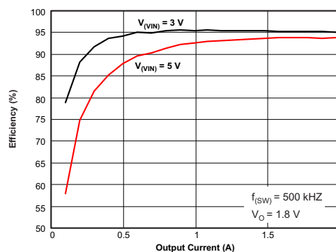
效率与输出电流间的关系
