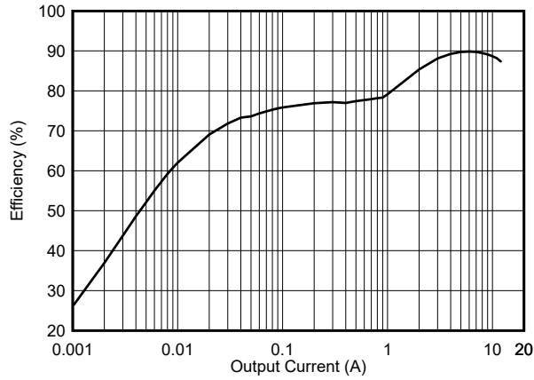
图 8-2. 效率
