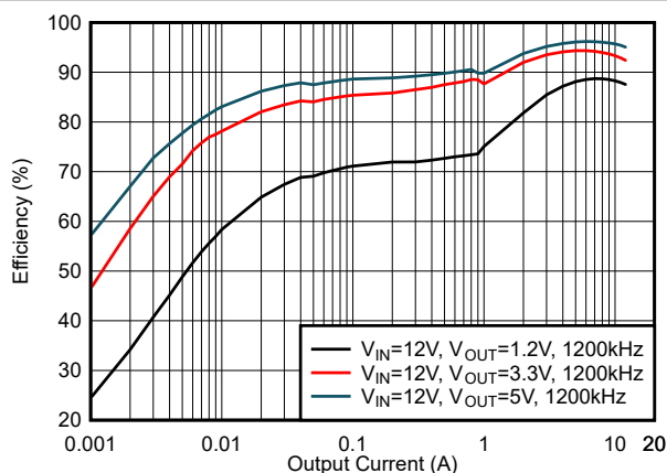
图 6-21. 效率, DCM 模式, f_{sw} = 1200\text{kHz}
