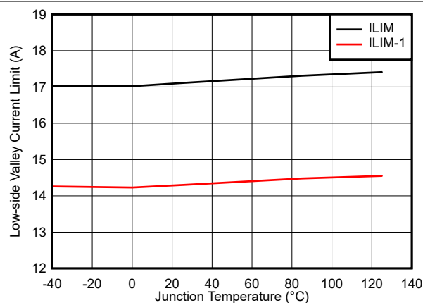
图 6-9. TPS56C231 电流限制与温度间的关系
