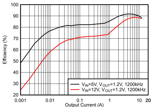
图 6-15. 效率, DCM 模式, f_{SW} = 1200\text{kHz}
