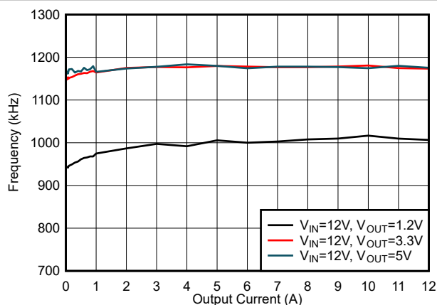
图 6-33. f_{SW} 负载调节, FCCM 模式, f_{SW} = 1200\text{kHz}
