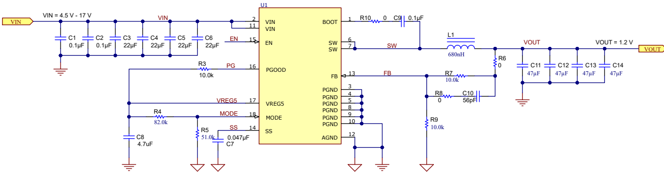
图 8-1. 应用原理图
