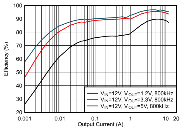
图 6-19. 效率, DCM 模式, f_{sw} = 800\text{kHz}
