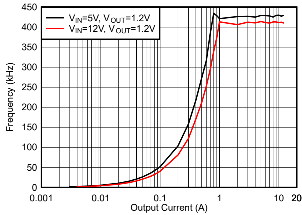
图 6-25. f_{SW} 负载调节, DCM 模式, f_{SW} = 400\text{kHz}
