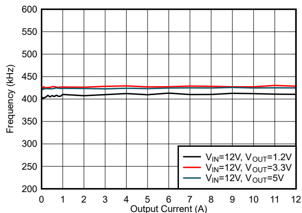
图 6-31. f_{SW} 负载调节, FCCM 模式, f_{SW} = 400\text{kHz}
