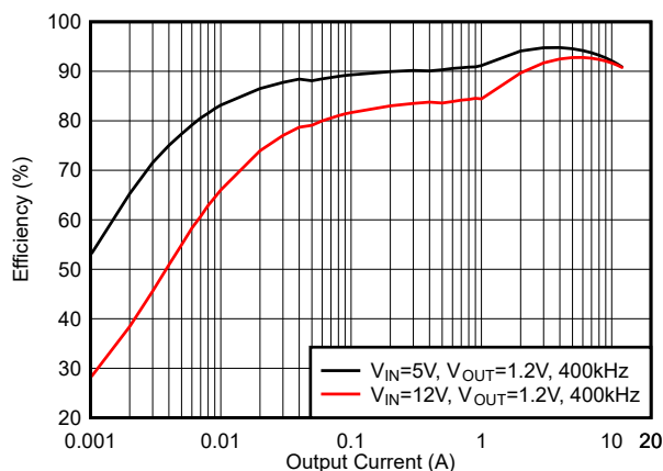
图 6-11. 效率, DCM 模式, f_{SW} = 400\text{kHz}
