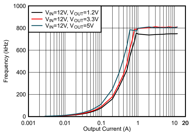
图 6-35. f_{SW} 负载调节, DCM 模式, f_{SW} = 800\text{kHz}
