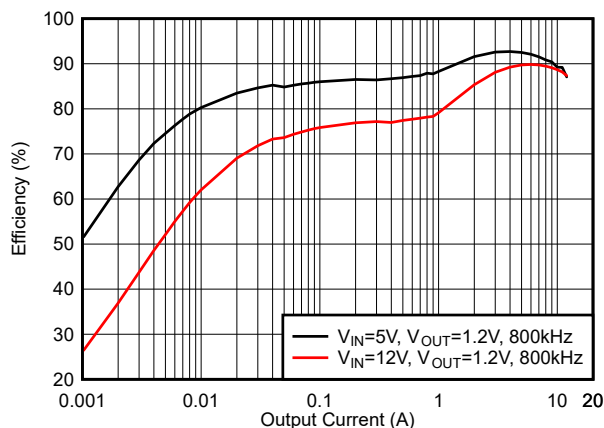
图 6-13. 效率, DCM 模式, f_{SW} = 800\text{kHz}
