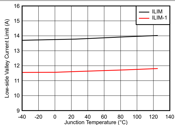
图 6-10. TPS56C231L 电流限制与温度间的关系
