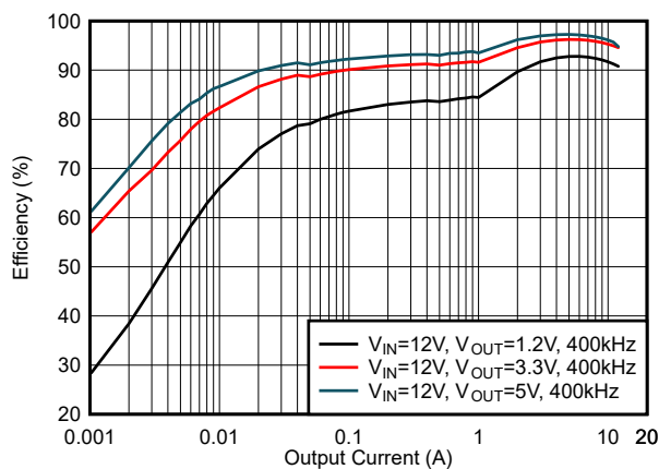
图 6-17. 效率, DCM 模式, f_{SW} = 400\text{kHz}
