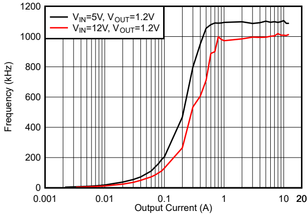
图 6-27. f_{SW} 负载调节, DCM 模式, f_{SW} = 1200\text{kHz}
