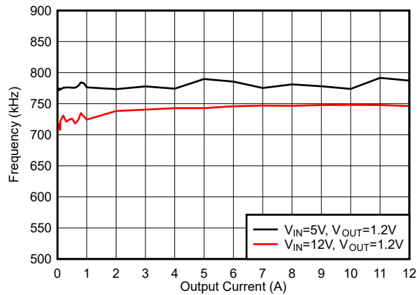
图 6-29. f_{SW} 负载调节, FCCM 模式, f_{SW} = 800\text{kHz}
