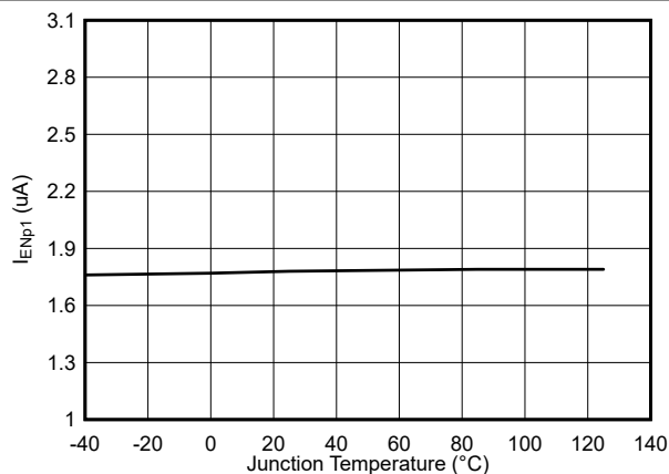
图 6-7. 使能上拉电流, V_{EN} = 1\text{V}
