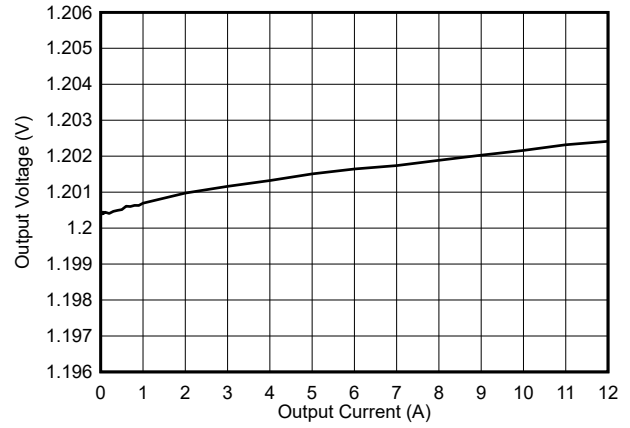
图 8-3. 负载调整率
