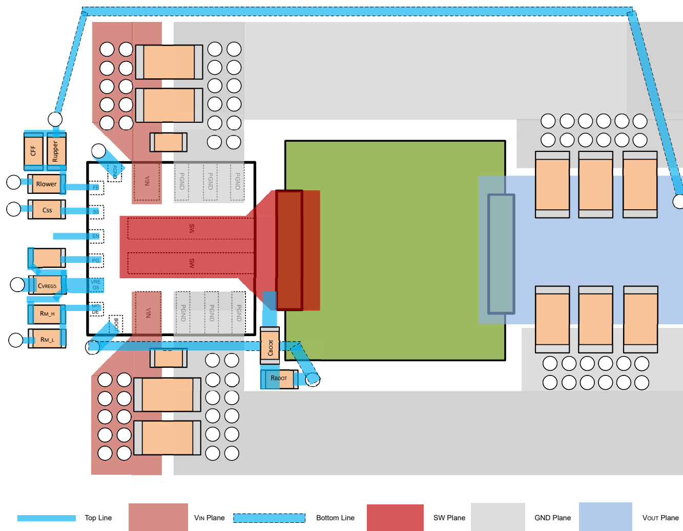
图 8-10. 布局示例
