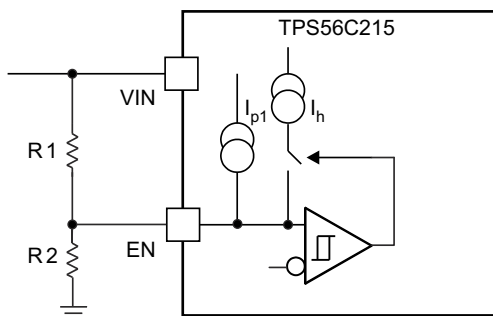
图 6-3. 可调节 VIN 欠压锁定
