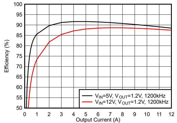
图 5-14. 效率, FCCM 模式, f_{sw} = 1200\text{kHz}
