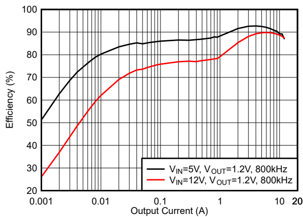
图 5-11. 效率, DCM 模式, f_{sw} = 800\text{kHz}
