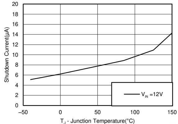
图 5-2. 关断电流与温度间的关系
