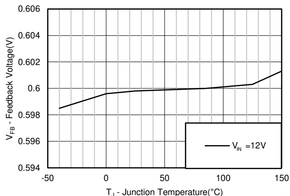
图 5-3. 反馈电压与温度之间的关系
