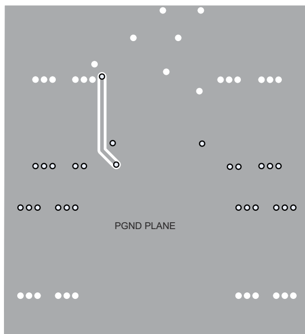
图 7-12. 底层布局
