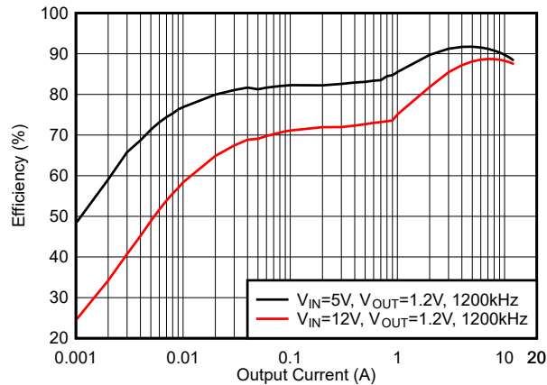
图 5-13. 效率, DCM 模式, f_{sw} = 1200\text{kHz}
