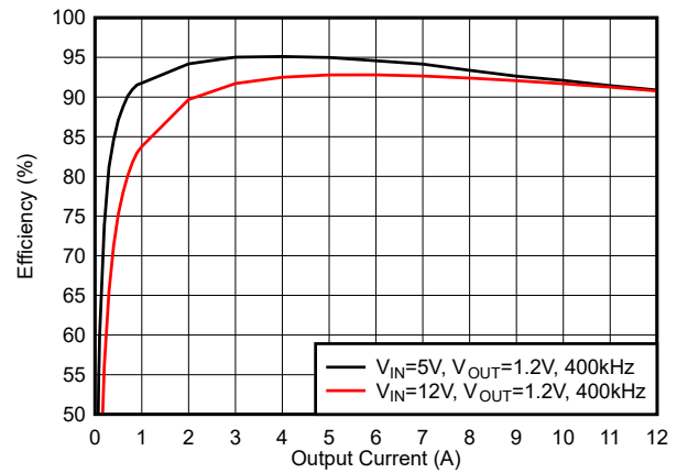
图 5-10. 效率, FCCM 模式, f_{sw} = 400\text{kHz}
