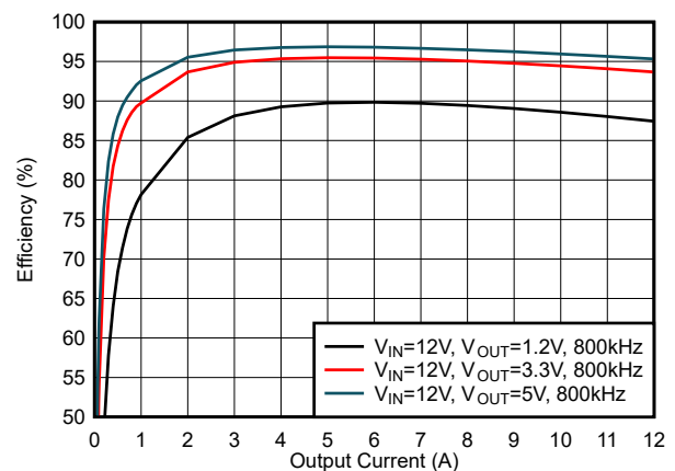
图 5-18. 效率, FCCM 模式, f_{sw} = 800\text{kHz}
