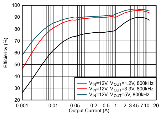
图 5-17. 效率, DCM 模式, f_{sw} = 800\text{kHz}
