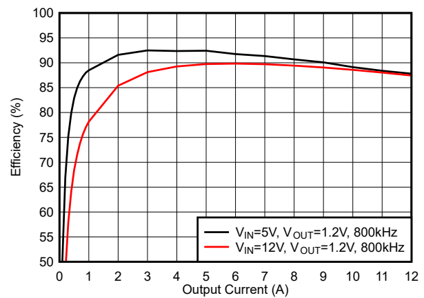
图 5-12. 效率, FCCM 模式, f_{sw} = 800\text{kHz}
