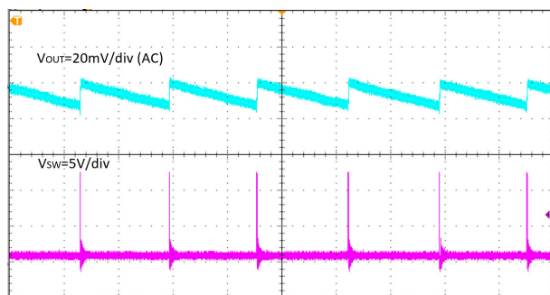
图 7-4. 输出电压纹波, I_{OUT} = 10mA , 时间 = 80 \mu s/div
