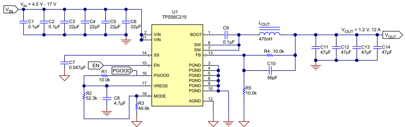
图 7-1. 应用原理图
