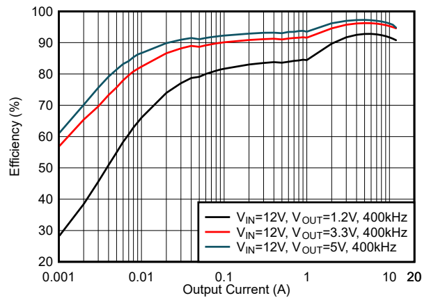
图 5-15. 效率, DCM 模式, f_{sw} = 400\text{kHz}
