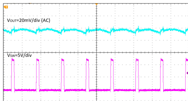
图 7-5. 输出电压纹波, I_{OUT} = 12A , 时间 = 1 \mu s/div
