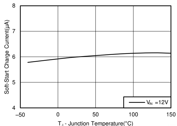
图 5-4. 软启动充电电流与温度间的关系
