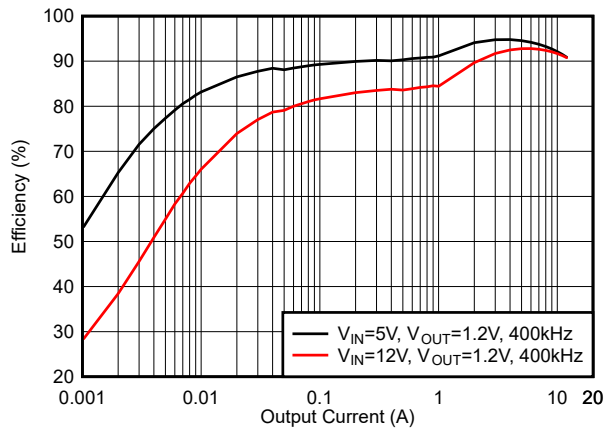
图 5-9. 效率, DCM 模式, f_{sw} = 400\text{kHz}
