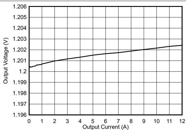
图 7-3. 负载调整率
