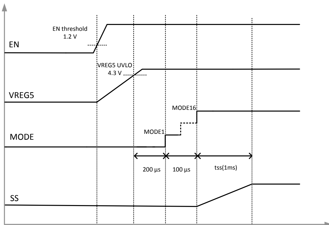
图 6-2. 上电序列
