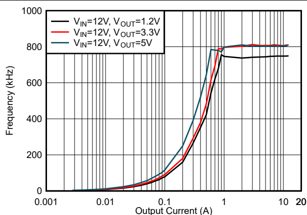
图 5-33. F_{SW} 负载调节, 模式 = DCM, F_{SW} = 800\text{kHz}
