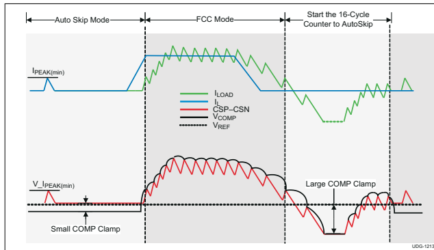
图 6-4. FCCM 瞬态响应
