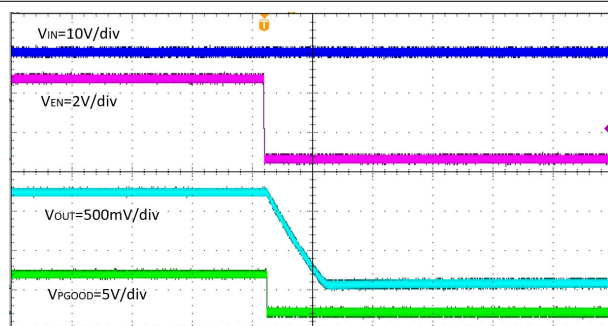
图 7-7. 相对于 EN 下降的关断, 时间 = 200 \mu s/div
