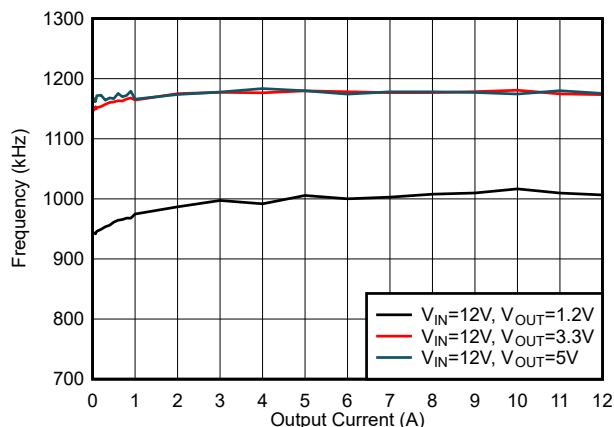
图 5-31. F_{SW} 负载调节, 模式 = FCCM, F_{SW} = 1200\text{kHz}
