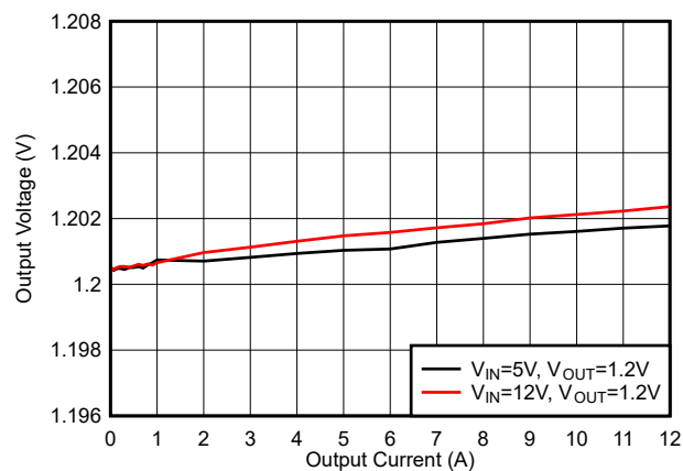
图 5-22. 负载调节, f_{sw} = 800\text{kHz}
