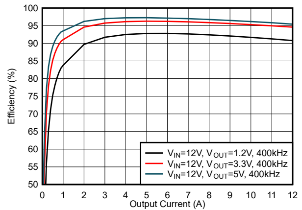
图 5-16. 效率, FCCM 模式, f_{sw} = 400\text{kHz}
