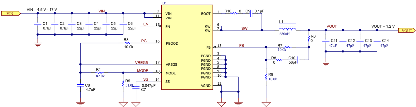
图 8-1. 应用原理图
