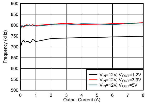
图 6-32. f_{SW} 负载调节, 模式 = FCCM, f_{SW} = 800kHz
