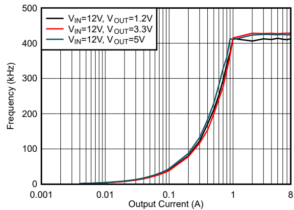
图 6-34. f_{SW} 负载调节, 模式 = DCM, f_{SW} = 400kHz
