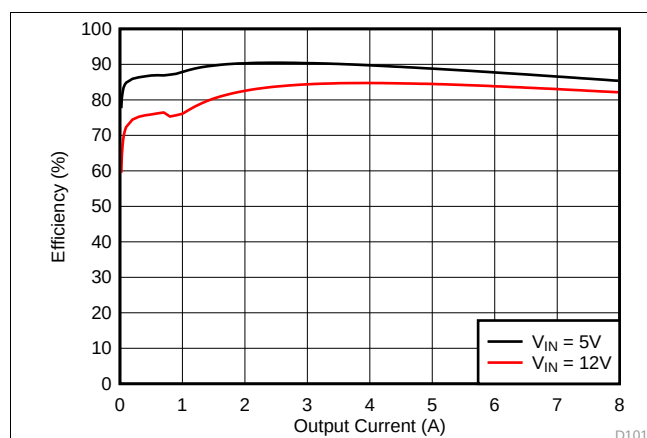
图 23. Efficiency
