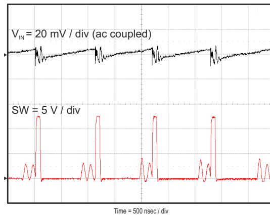
图 8-9. Input Voltage Ripple, I_{OUT} = 700 mA
