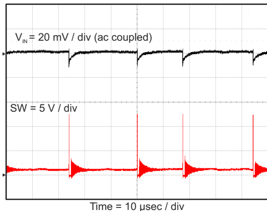
图 8-8. Input Voltage Ripple, I_{OUT} = 10 mA
