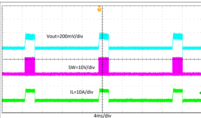
图 8-21. 输出硬短路断续
