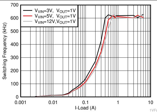
图 7-6. TPS566231 F_{SW} vs Output Load
