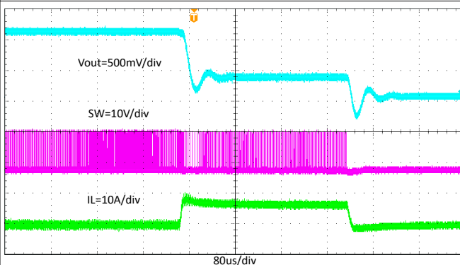
图 8-19. TPS565242 正常运行至输出硬短路
