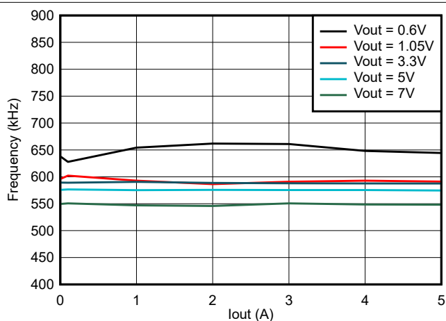
图 6-9. TPS565242 频率与负载间的关系
