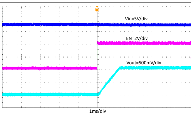
图 8-15. 通过 EN 启动, I_{OUT} = 5A
