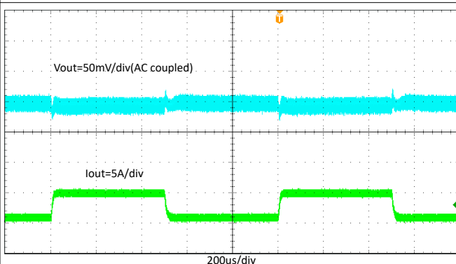
图 8-11. TPS565242 瞬态响应, 0.5A 至 4.5A, 负载阶跃为 2.5A/ \mu s
