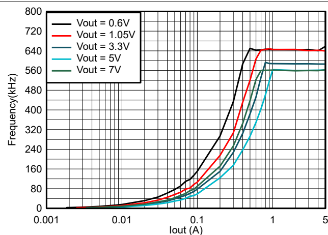
图 6-10. TPS565242 频率与负载间的关系
