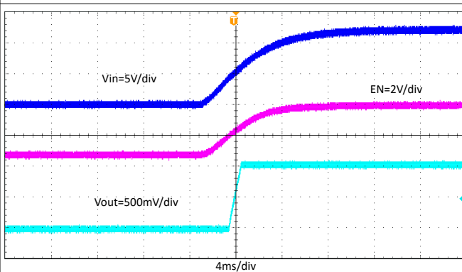
图 8-17. 在 V_{IN} 上升时启动, I_{OUT} = 5A
