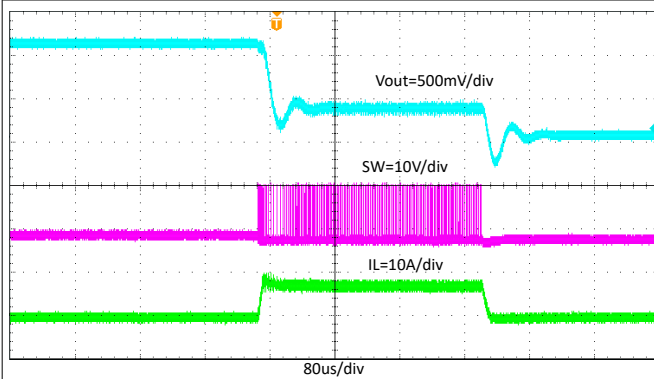
图 8-20. TPS565247 正常运行至输出硬短路
