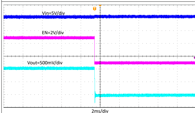
图 8-16. 通过 EN 关断, I_{OUT} = 5A
