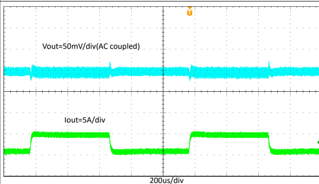
图 8-13. TPS565247 瞬态响应, 0.5A 至 4.5A, 负载阶跃为 2.5A/ \mu s
