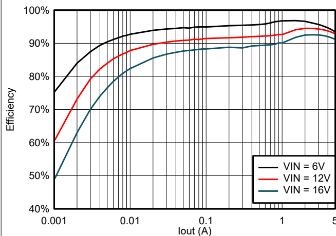
图 6-15. TPS565242 在 3.3V OUT 且使用 2.2 \mu H 电感器时的效率
