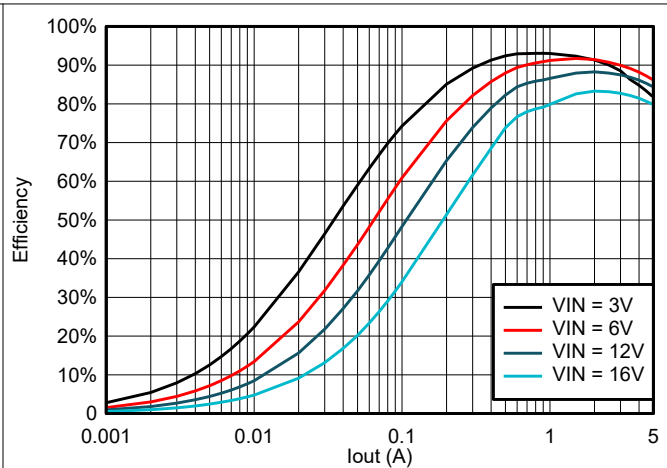
图 6-14. TPS565247 在 1.05V OUT 且使用 1 \mu H 电感器时的效率
