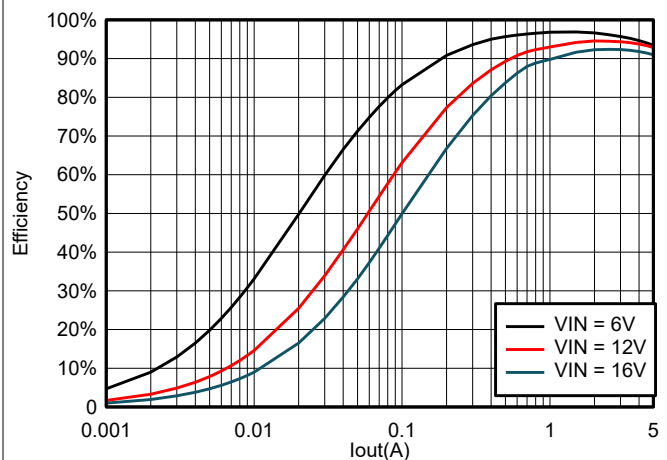
图 6-16. TPS565247 在 3.3V OUT 且使用 2.2 \mu H 电感器时的效率
