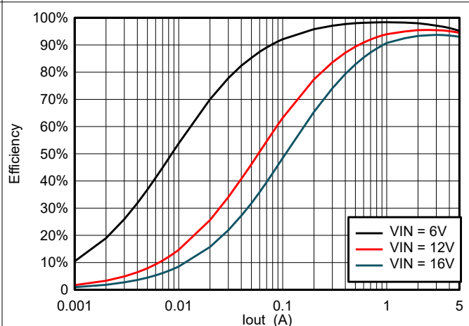
图 6-18. TPS565247 在 5V OUT 且使用 2.2 \mu H 电感器时的效率
