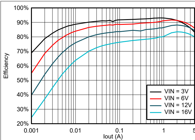
图 6-13. TPS565242 在 1.05V OUT 且使用 1 \mu H 电感器时的效率
