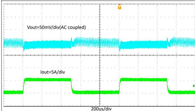
图 8-12. TPS565242 瞬态响应, 0.1A 至 5A, 负载阶跃为 2.5A/ \mu s
