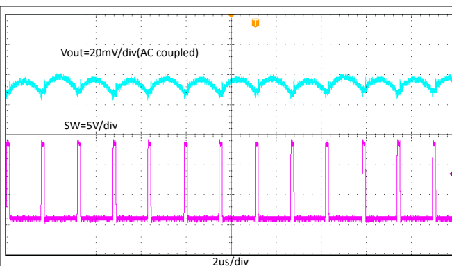
图 8-9. TPS565247 输出电压纹波 ( 0.01A 负载 )
