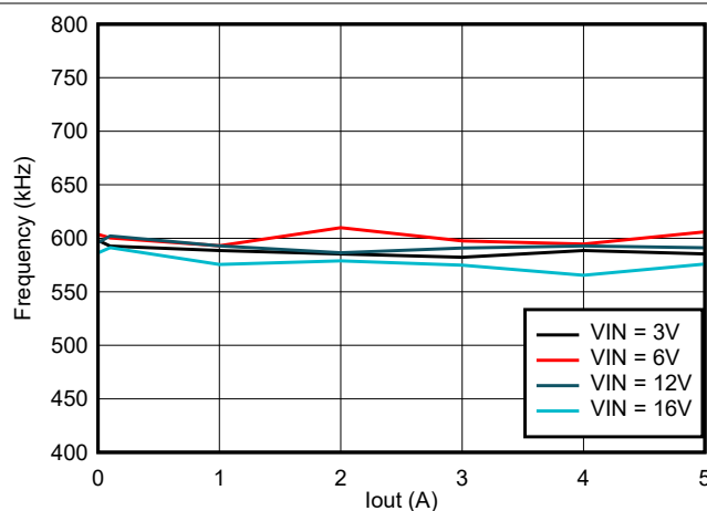
图 8-3. TPS565247 频率与负载间的关系
