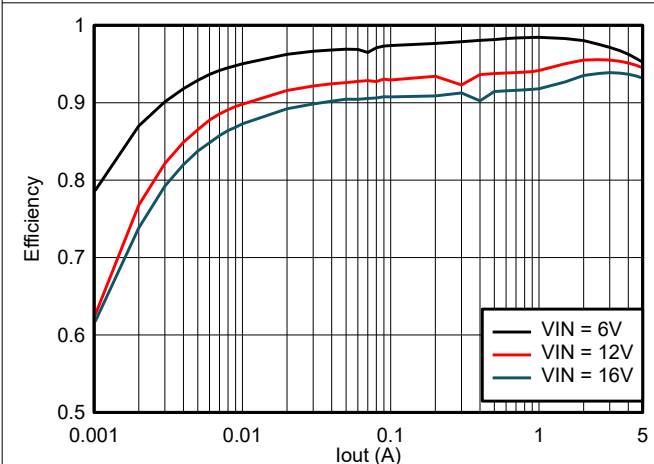
图 6-17. TPS565242 在 5V OUT 且使用 2.2 \mu H 电感器时的效率
