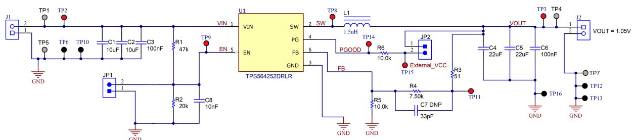
图 8-1. Schematic
